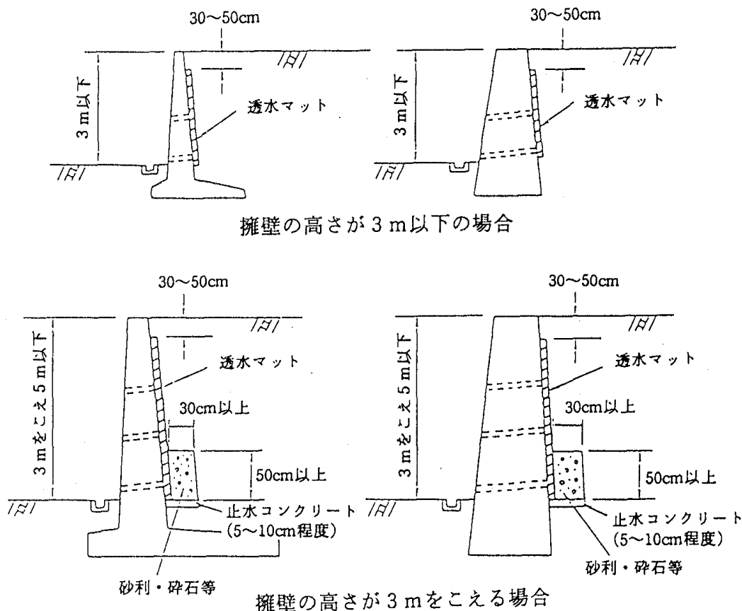
図7 擁壁高さ別施工形態
