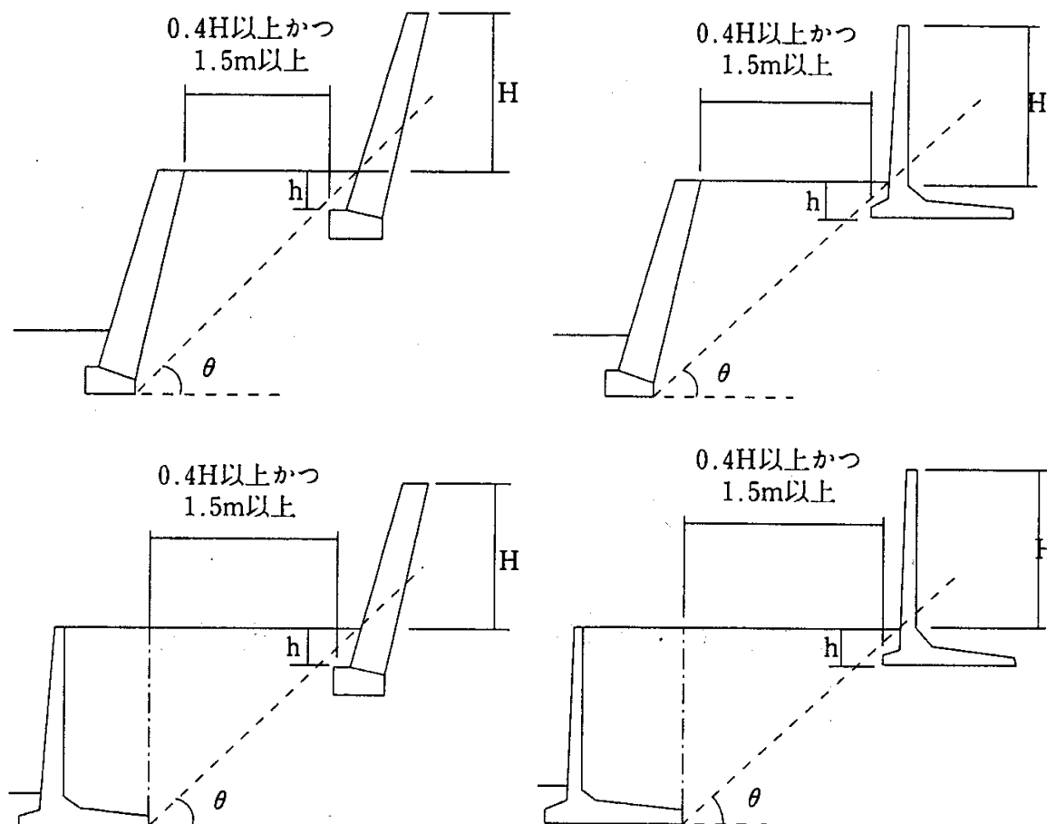
図13 上部・下部擁壁を近接して設置する場合
