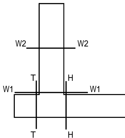
図5 応力度の照査位置(例)
