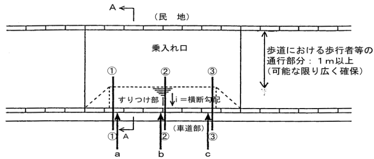
A-A断面
