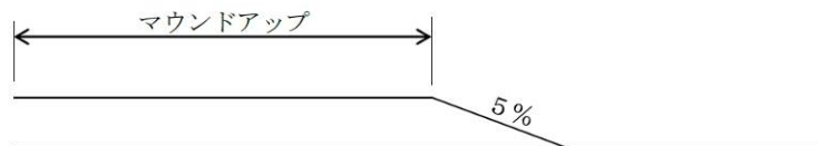
図3-10 マウントアップ歩道の摺付
