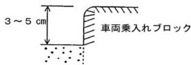
図3-2 縁石工(車両乗入れブロック)測定箇所
