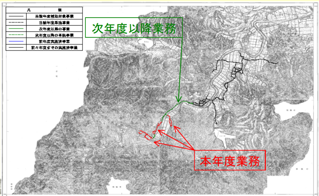
全体計画平面図－2(矢下付近)
