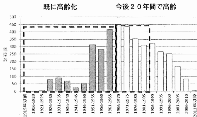
橋梁の建設年度別 分布
