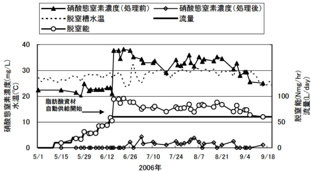
図4 浄化装置の処理条件及び処理能力(2006)
