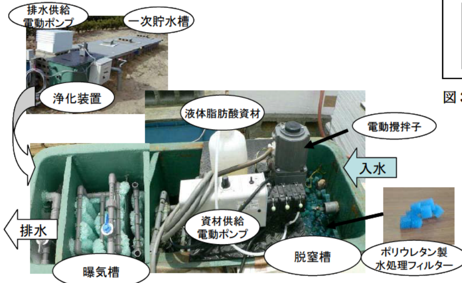
図2 浄化装置の構成
