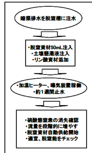
図3 浄化装置稼働手順
