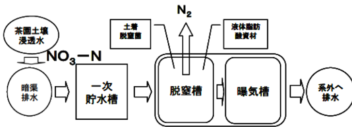
図1 茶園浸透水の浄化処理フロー
