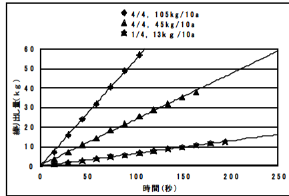
図3 時間経過と繰り出し量の関係
