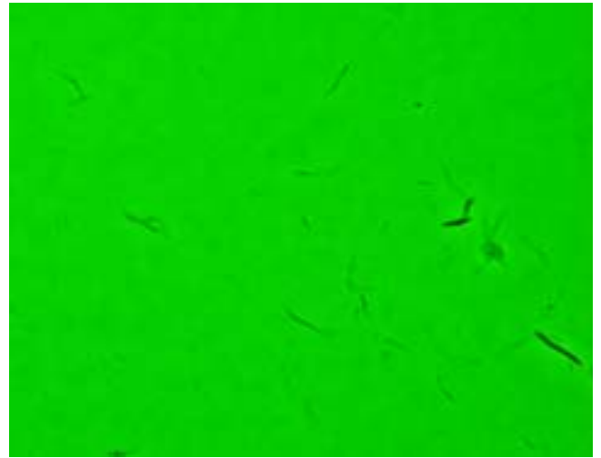
図2 アスベスト(クリソタイル)の位相差顕微鏡像 アスベストの微小な繊維はほとんど無色であり、通常の光学顕微鏡では判別が困難であるが、無色透明でも、光の位相の変化により位相差顕微鏡では明瞭に捉えることができる。
