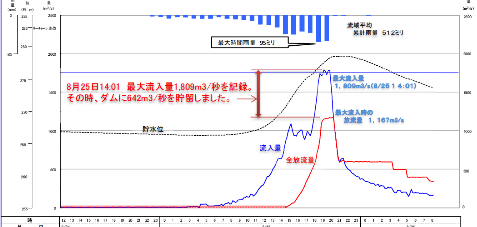
宮川ダム洪水調節記録図 (原因: 台風15号) (No. 1)
