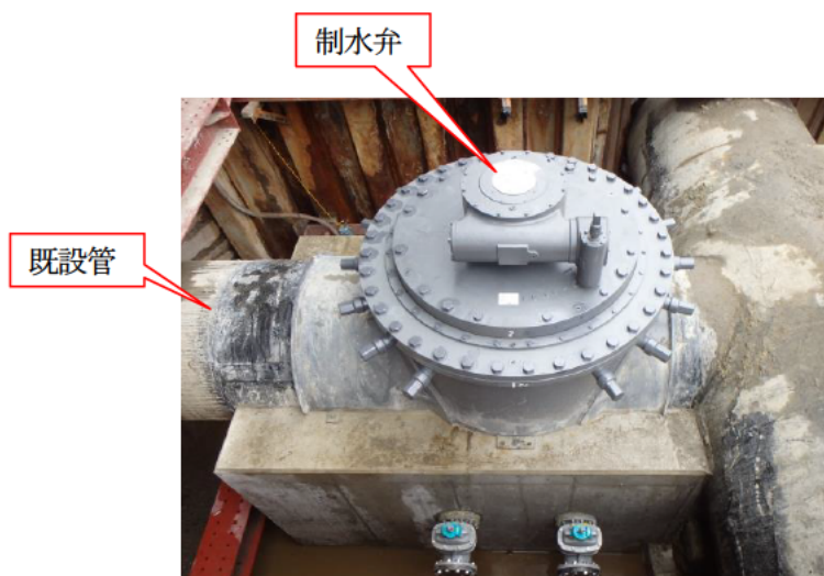
不断水工法による制水弁の設置状況 〔内径1350耗制水弁取替工事（四期・下深谷部）〕
