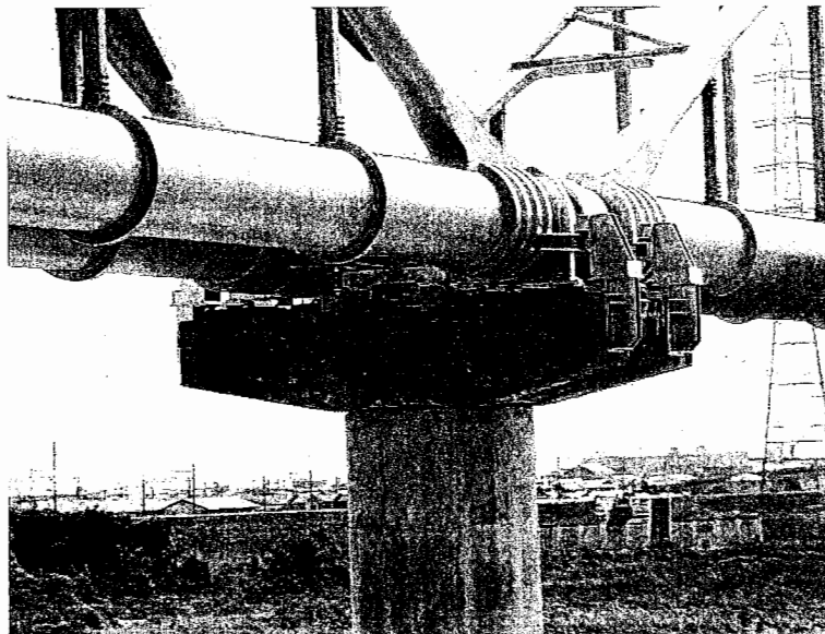
鈴鹿川第2水管橋の耐震補強
