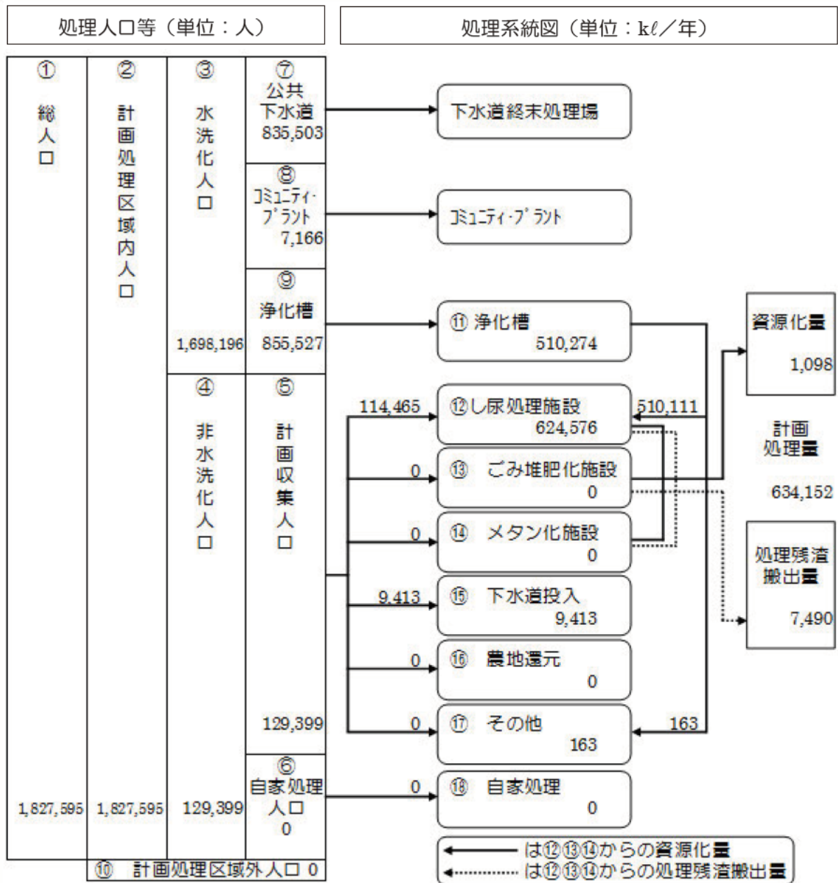
資料7-11 し尿処理のフロー図（平成26年度）
