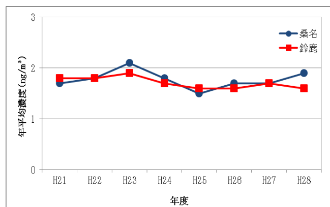
図 1 三重県における大気環境中の水銀濃度（年平均値）の推移
