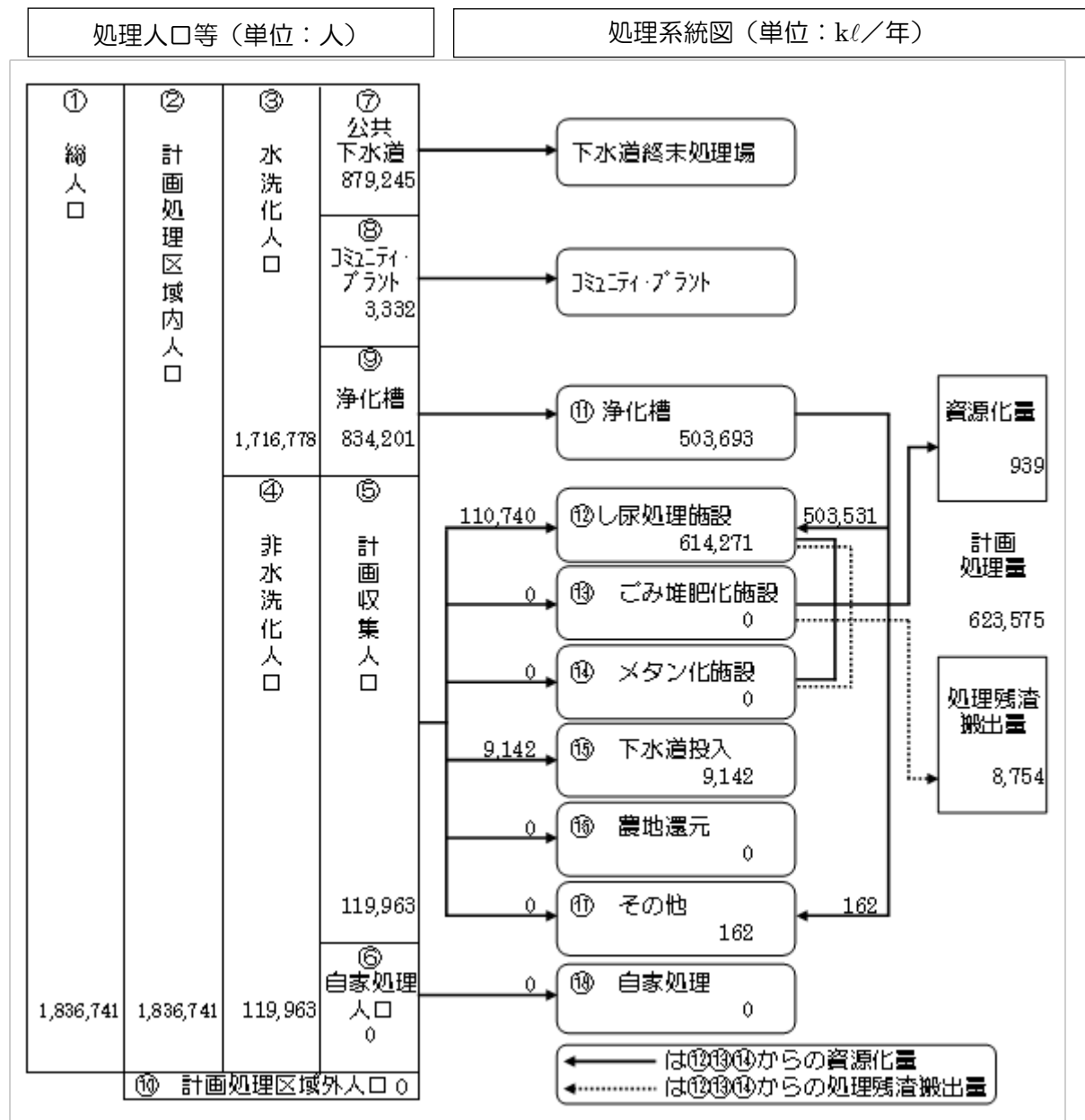
資料7-11 し尿処理のフロー図（平成27年度）
