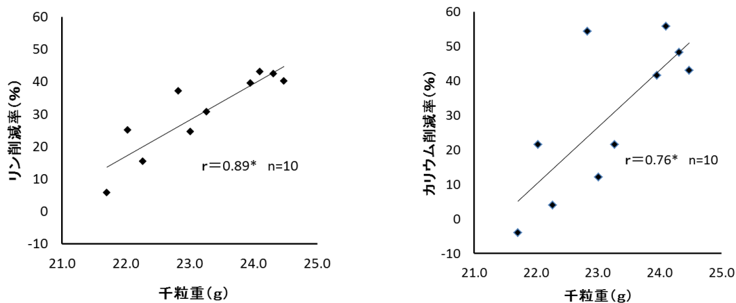
図1 玄米千粒重と高精白時(精米歩合 83%)のリン・カリウム削減率の関係 削減率は七訂日本食品標準成分表 精白米(水稻穀粒)の値に対する数値 千粒重は含水率 15%換算値。なお、供試サンプルは、異なる移植時期及び施肥条件で栽培し、 成熟期(出穂後 30-35 日)に収穫後、乾燥調製(1.85mm 粒選別)を行った。 *は 5%水準で有意であることを示す。
