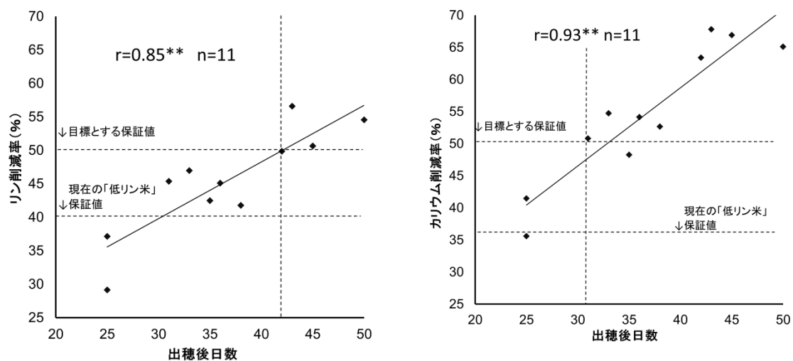
図2 刈取り時期(出穂後日数)と高精白時(精米歩合 83%)のリン・カリウム削減率の関係 出穂後 25 日からおよそ 3 日ごとに 50 日目まで複数回刈取り、登熟度合いの異なる玄米を収集 した。収穫後、乾燥調製(1.85mm 粒選別)した。 削減率は七訂日本食品標準成分表 精白米(水稻穀粒)の値に対する数値。 **は 1%水準で有意であることを示す。
