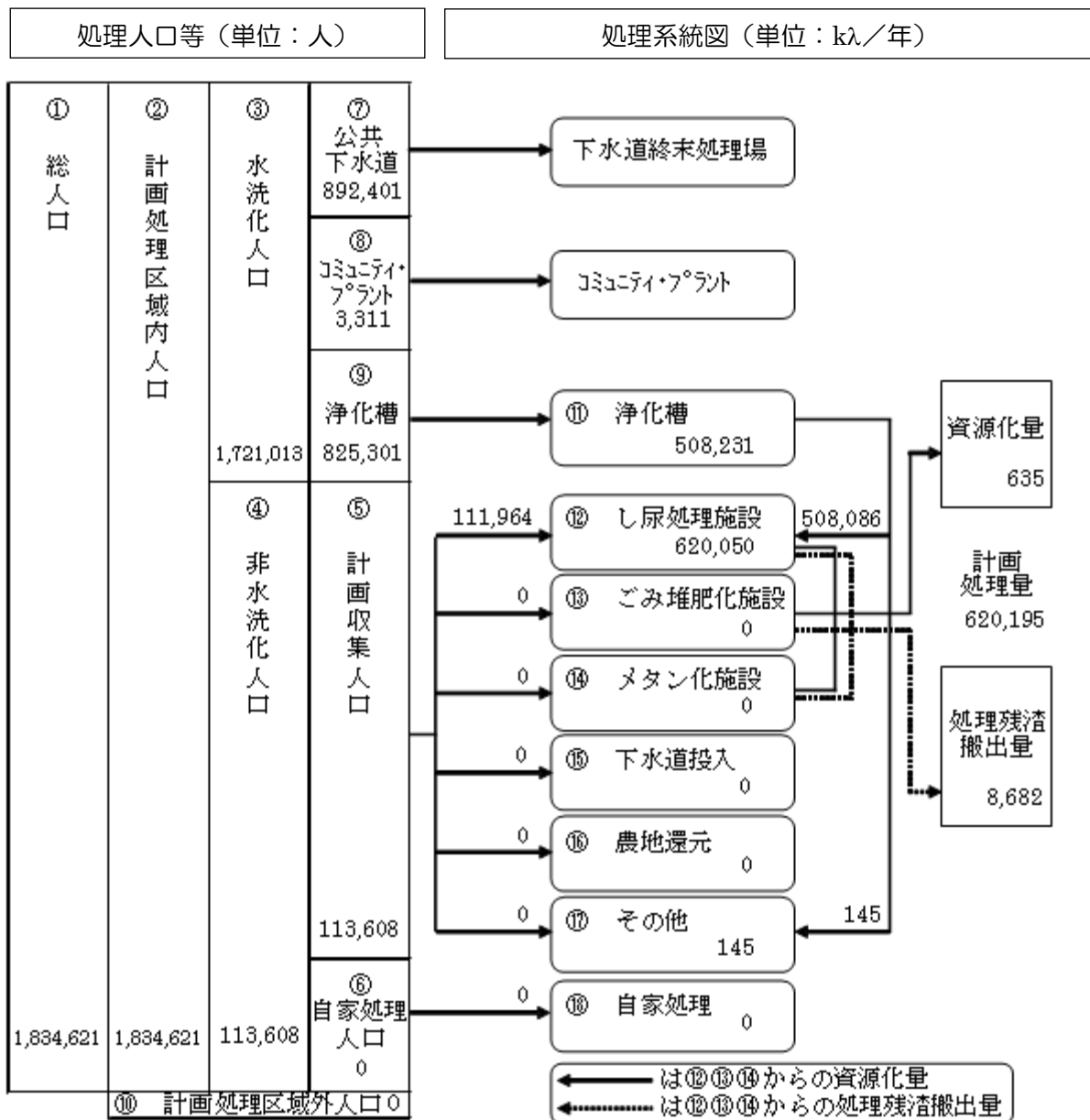
資料7-11 し尿処理のフロー図（平成28年度）
