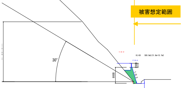
標準断面図 (Standard Cross-section Diagram)
