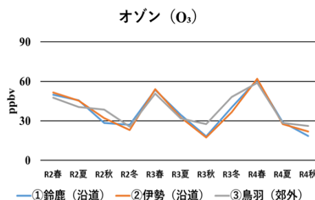
図5 オゾン濃度の季節変動
