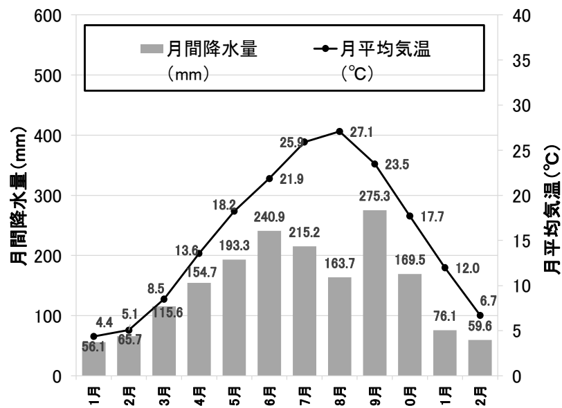
四日市市における月別平均気温、降水量 (気象庁四日市観測所 H26～R5の10カ年平均)
