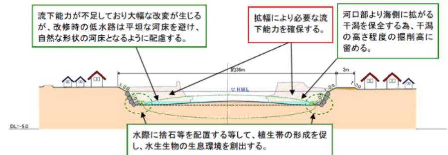
横断イメージ図(百々川)
