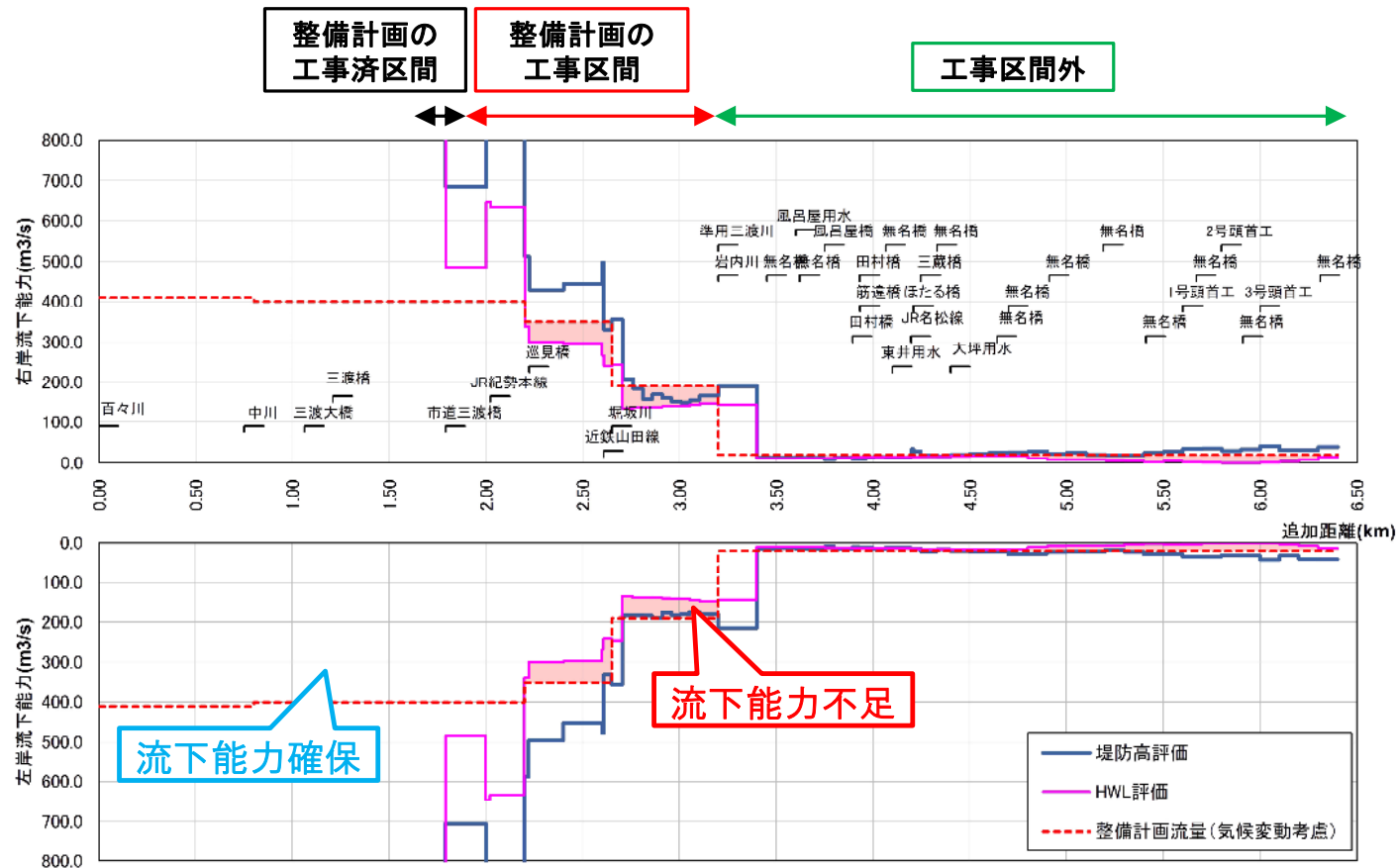
現況流下能力図(三渡川)
