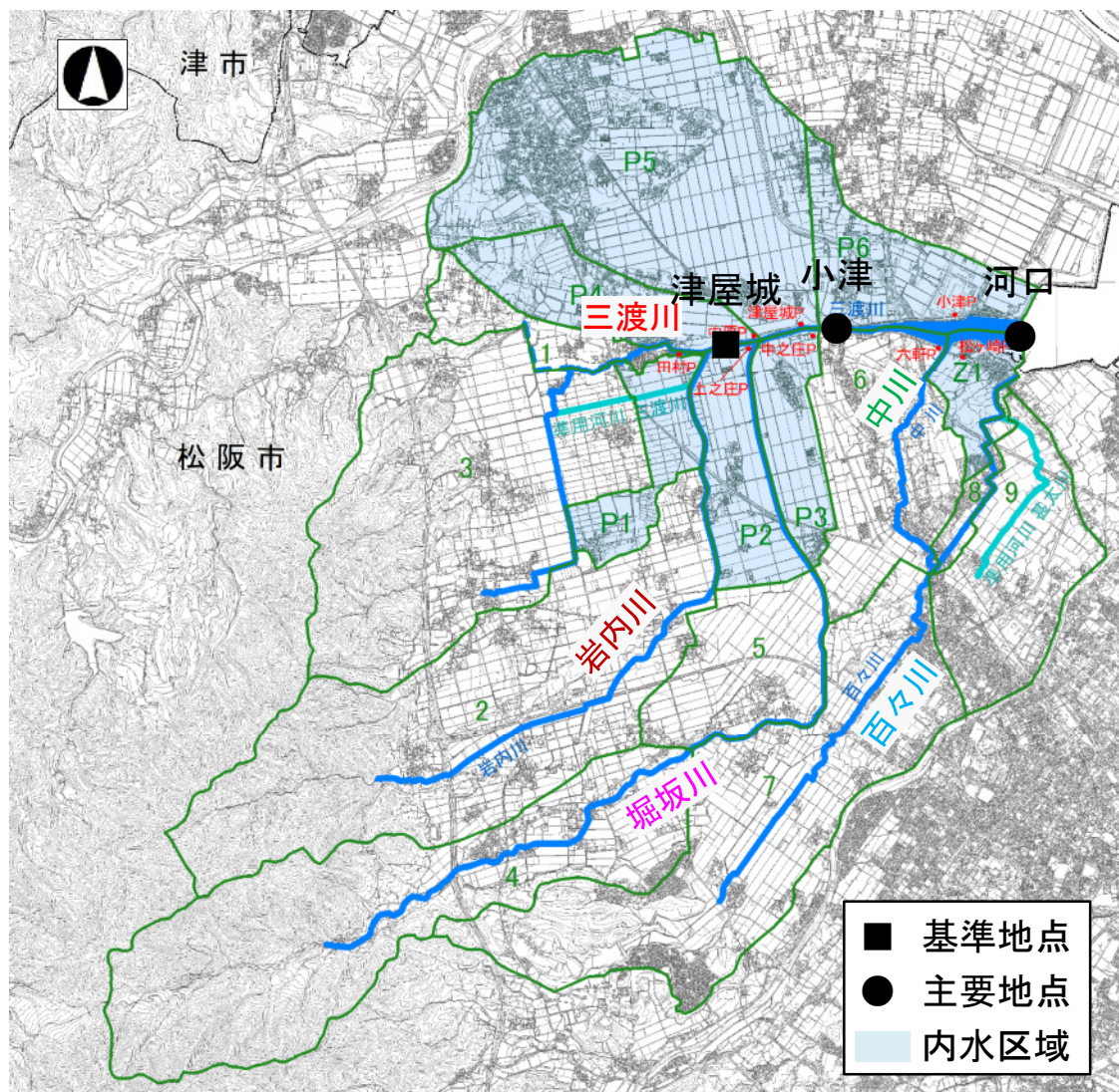
流域分割図(計画高水流量)
