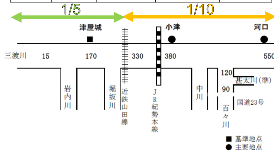
図 3-1：流量配分図
