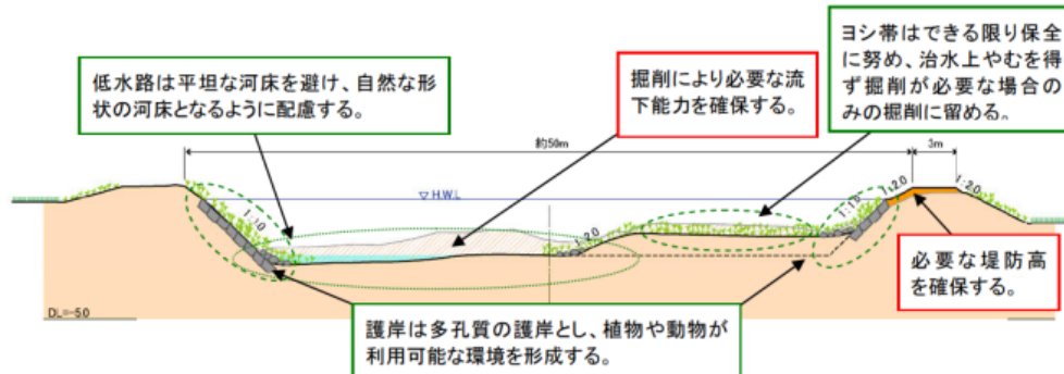
横断イメージ図(三渡川)
