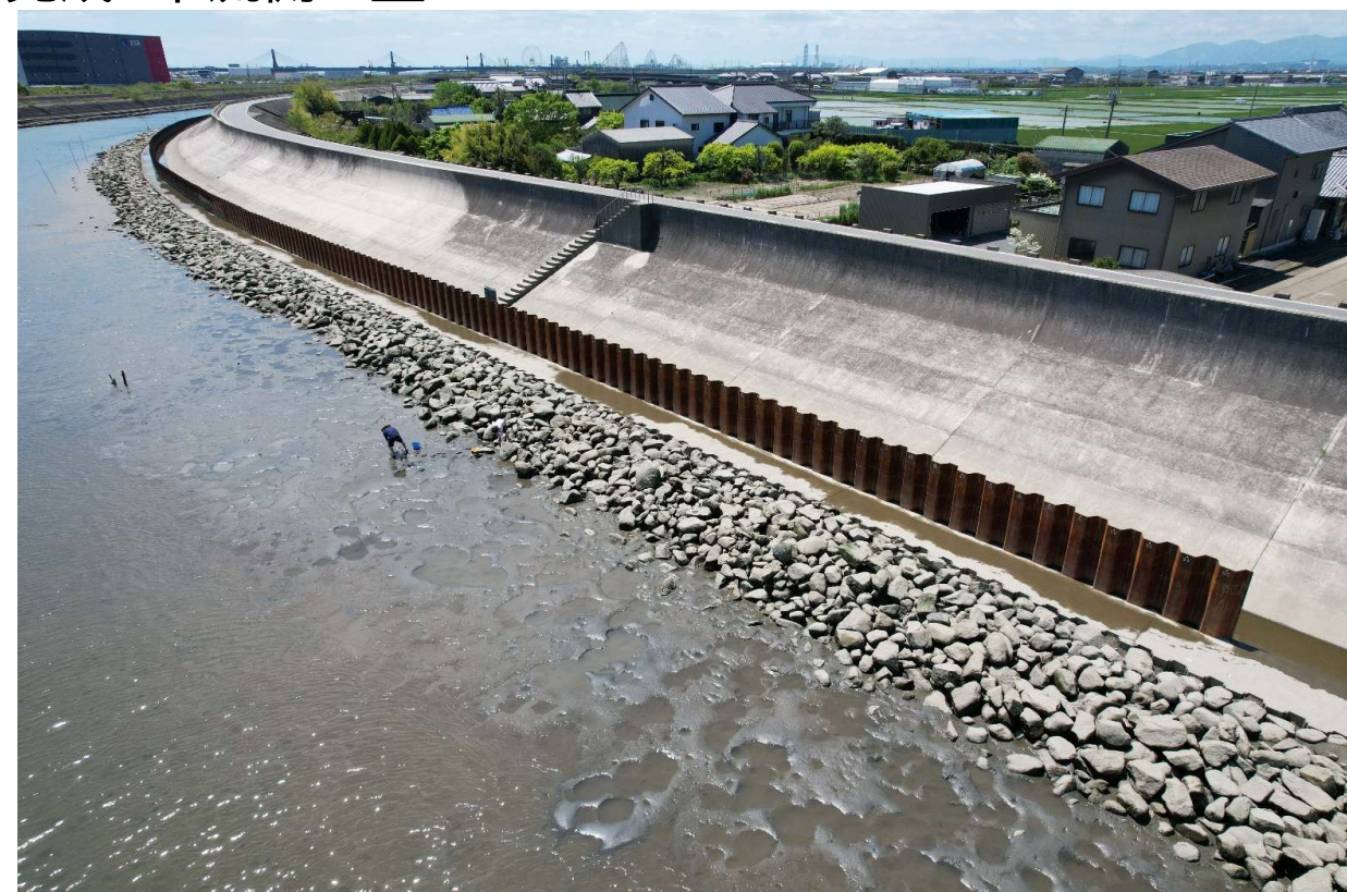
完成 下流側を望む
