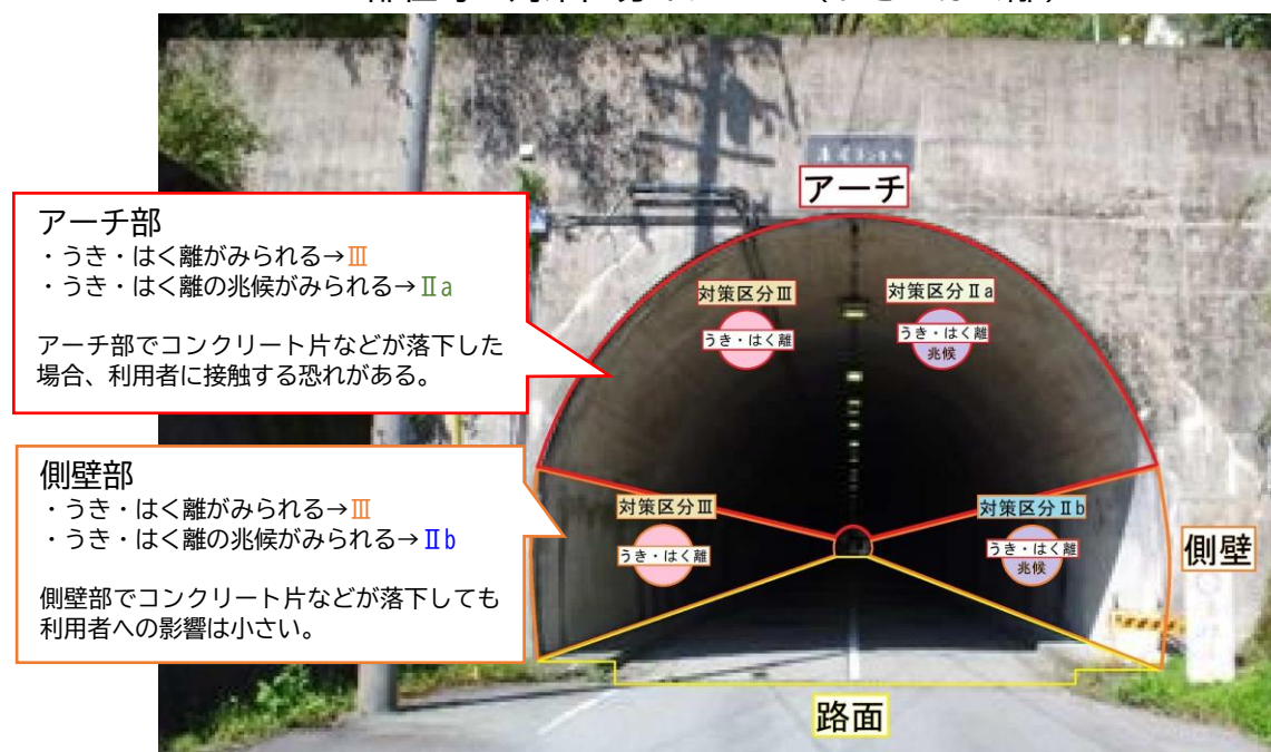
部位毎の対策区分イメージ（うき・はく離）
