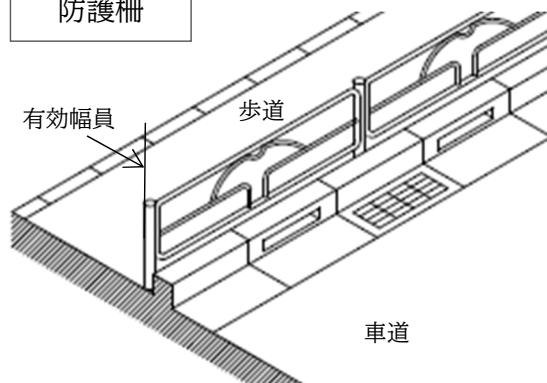
防護柵
