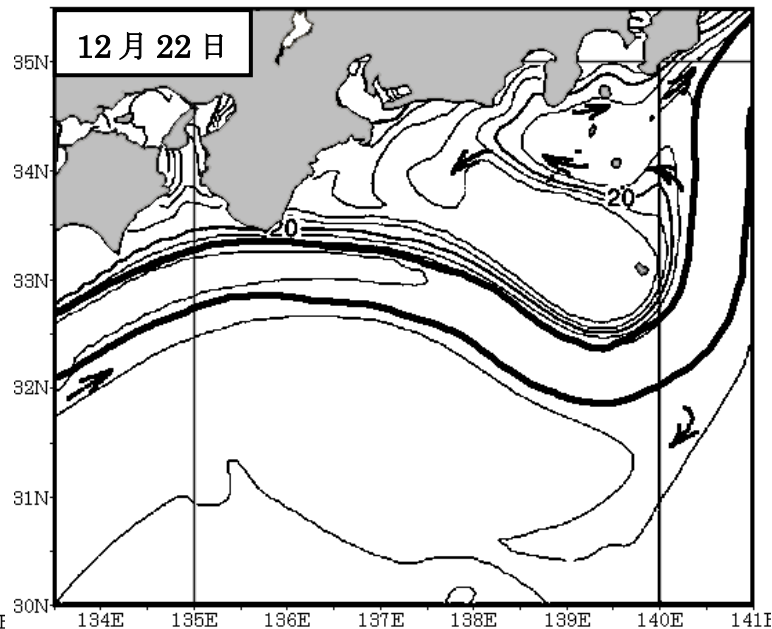
2025/12/22 気象庁 海面水温予想図より [表面水温]
