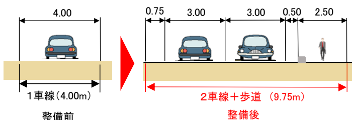
【標準断面図】
