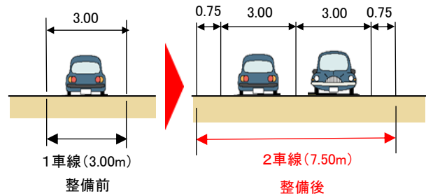
【標準断面図】
