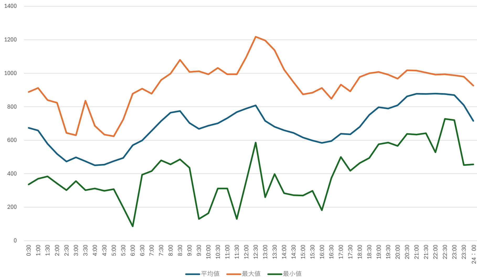
高野浄水場 受電電力量トレンド（9月）
