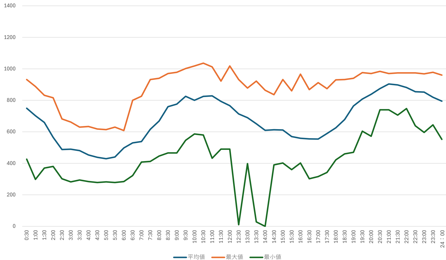
高野浄水場 受電電力量トレンド（11月）
