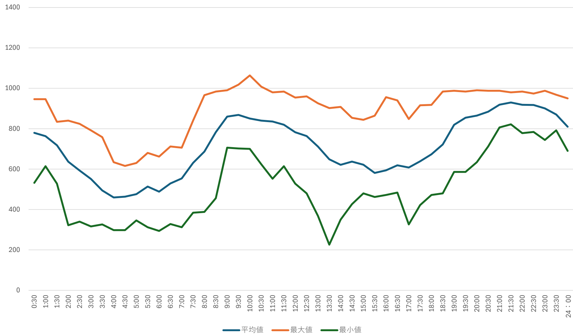
高野浄水場 受電電力量トレンド（3月）
