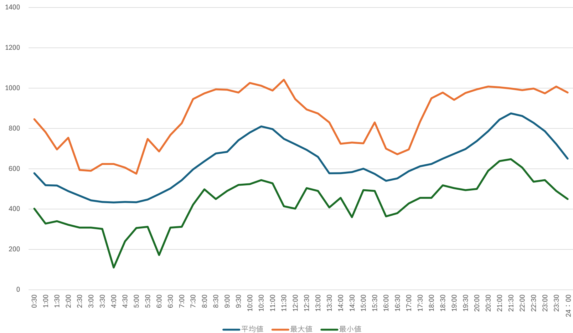
高野浄水場 受電電力量トレンド（8月）
