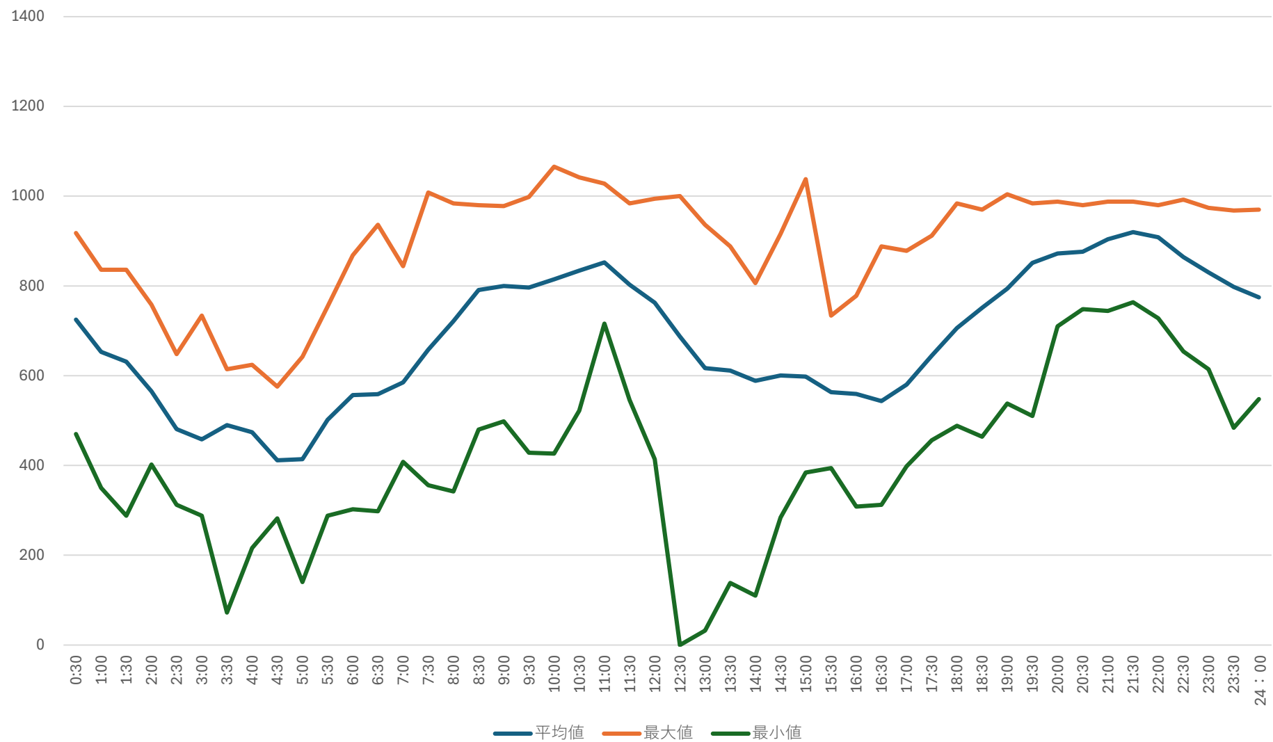
高野浄水場 受電電力量トレンド（10月）
