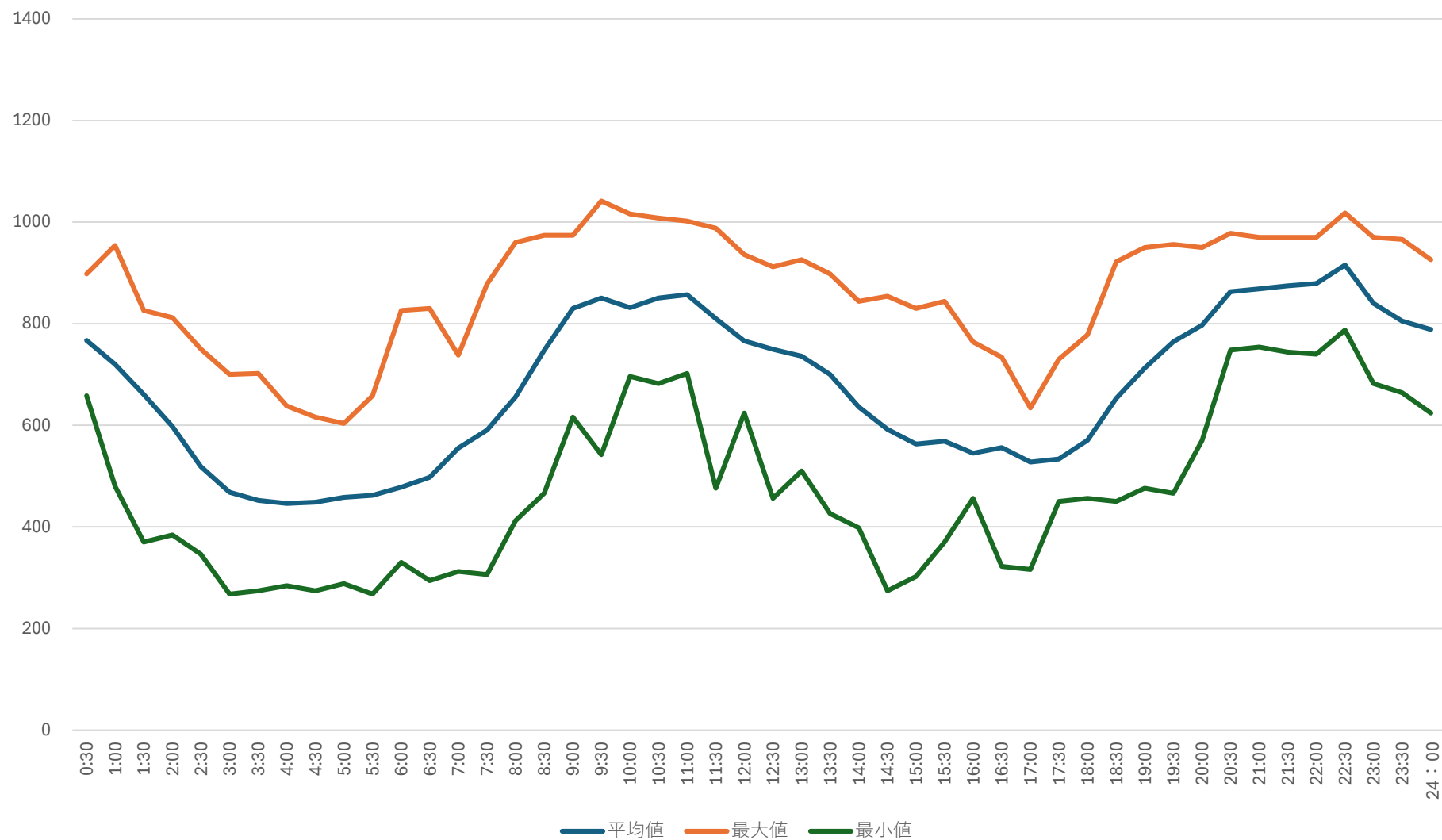
高野浄水場 受電電力量 トレンド（5月）
