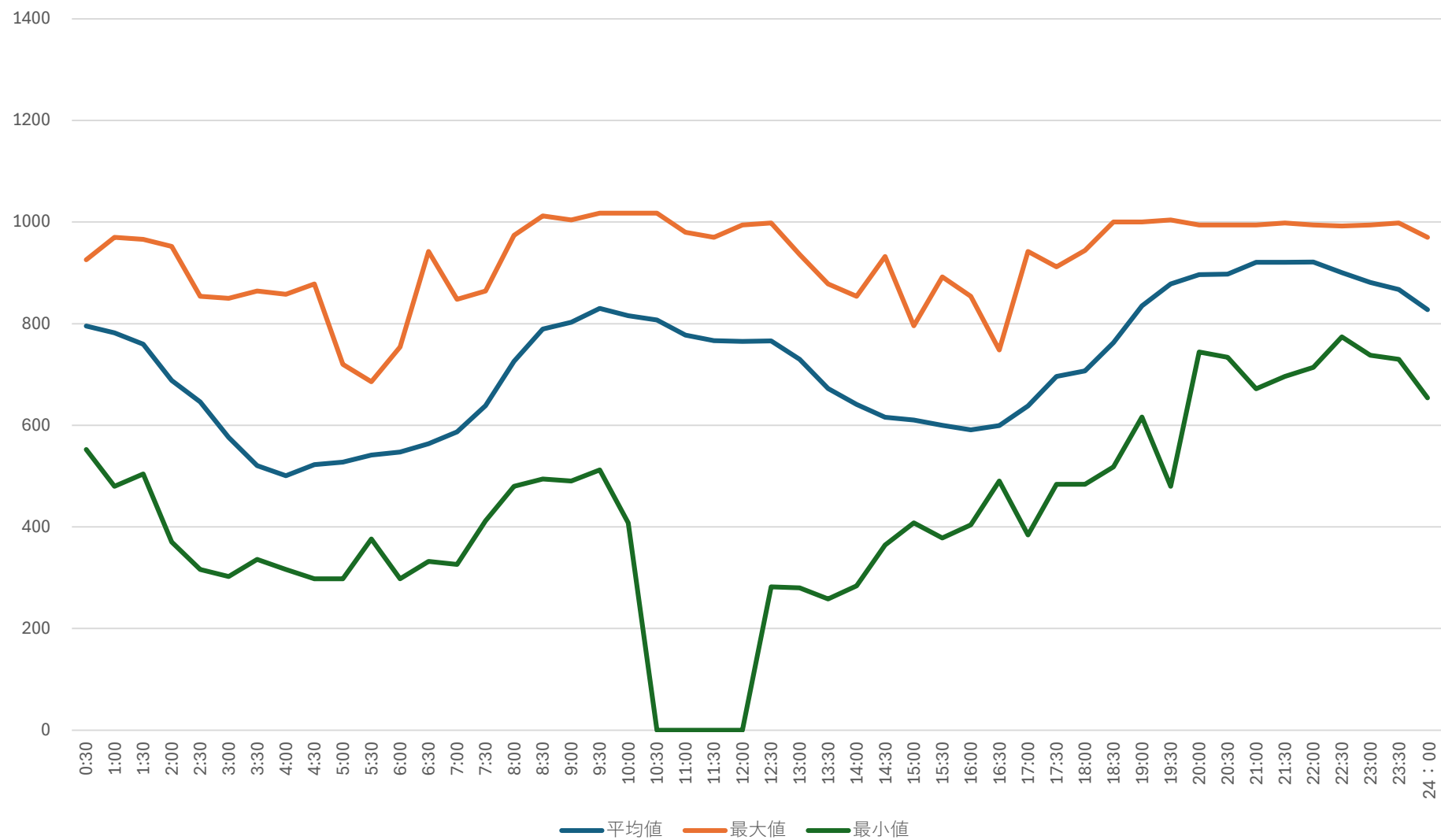
高野浄水場 受電電力量トレンド（1月）
