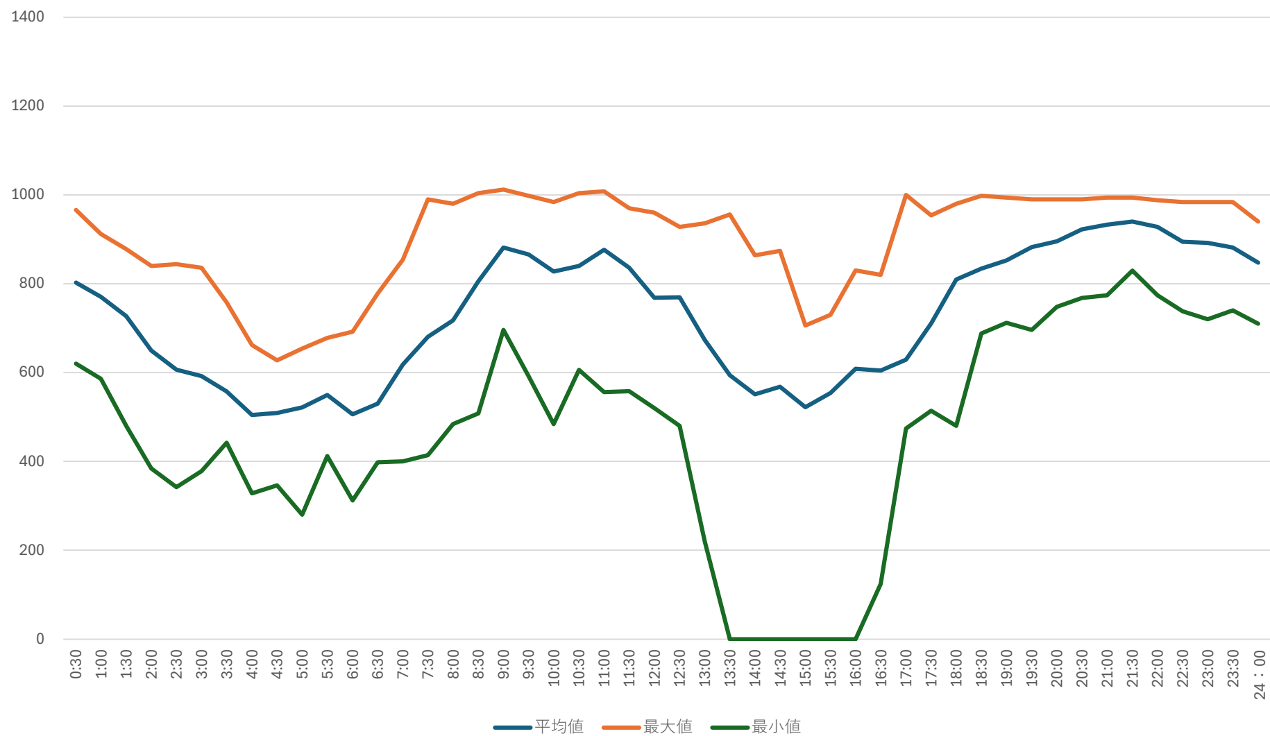
高野浄水場 受電電力量トレンド（2月）
