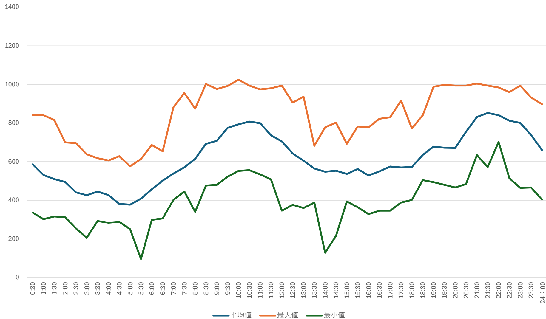
高野浄水場 受電電力量トレンド（7月）
