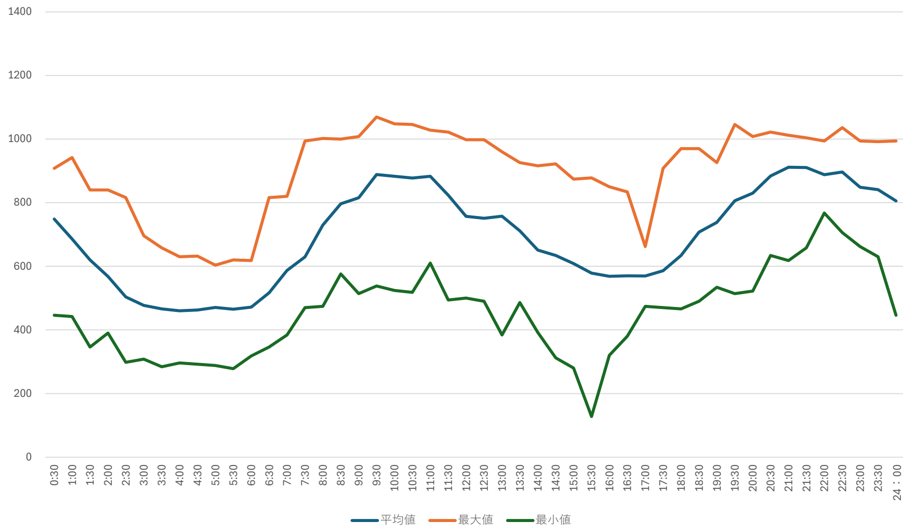
高野浄水場 受電電力量 トレンド（6月）
