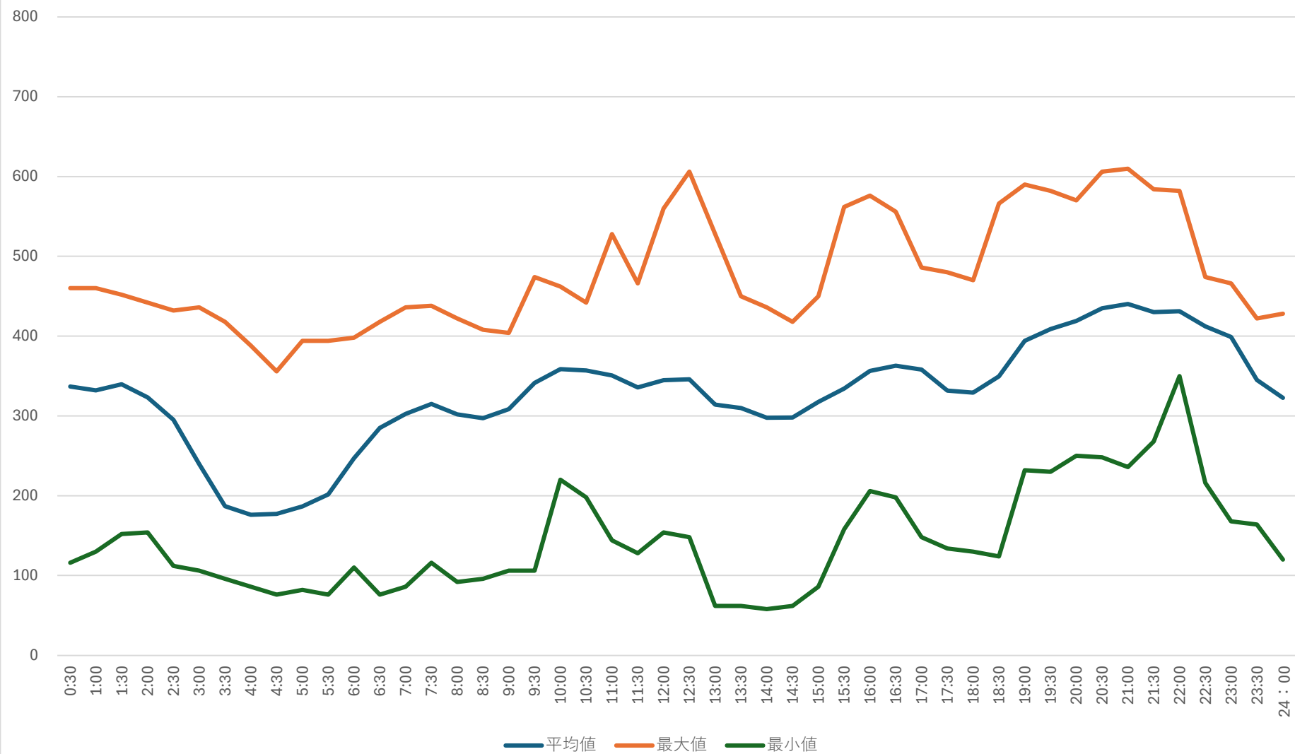
大里浄水場 受電電力量トレンド（1月）
