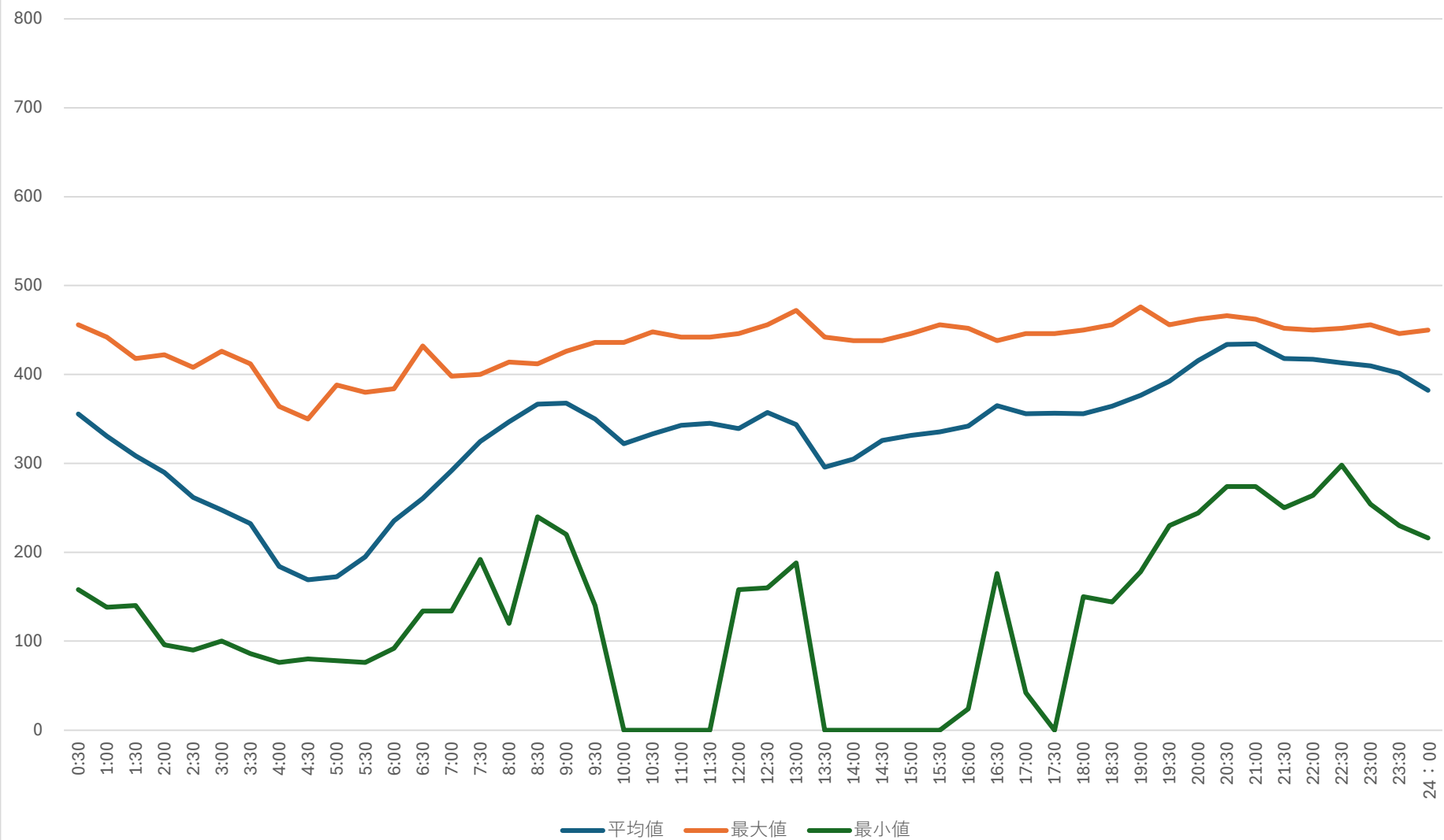
大里浄水場 受電電力量トレンド（10月）
