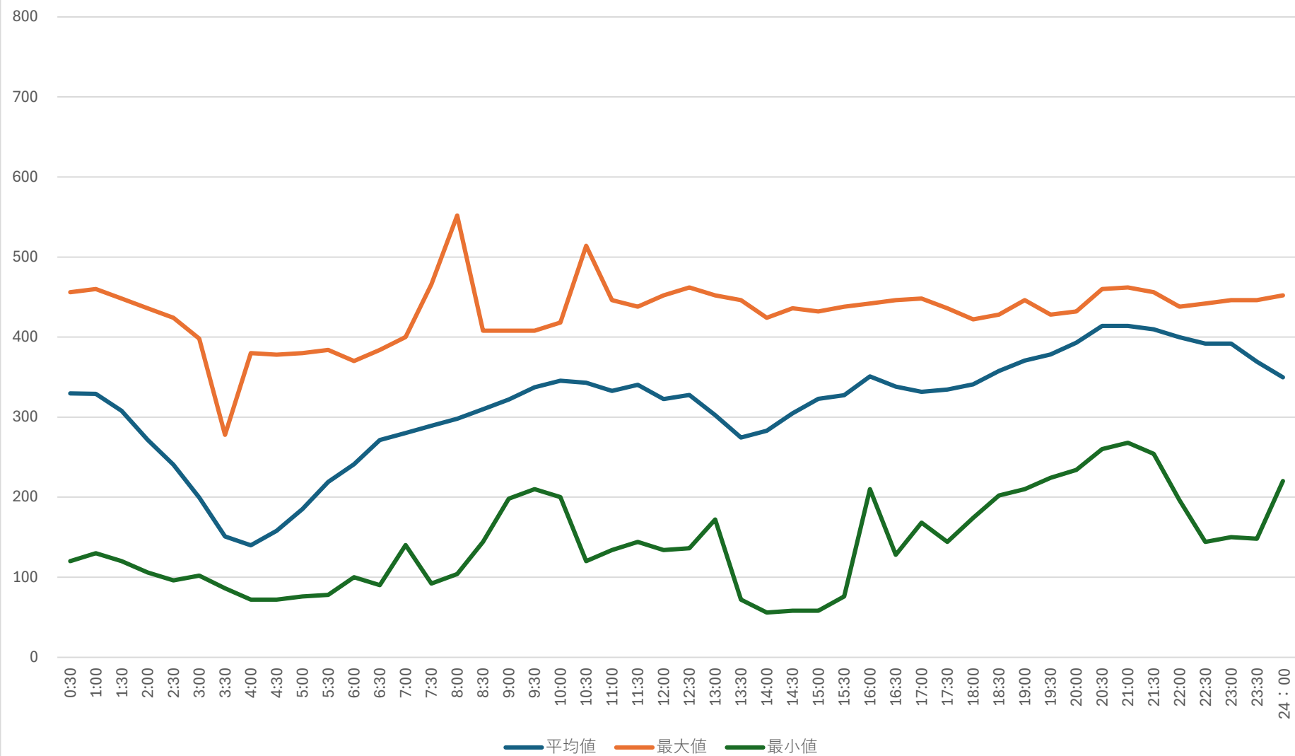
大里浄水場 受電電力量トレンド（2月）
