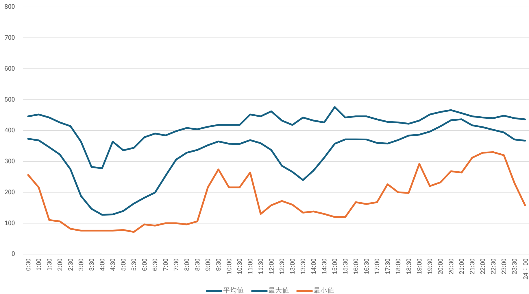
大里浄水場 電力量トレンド（5月）
