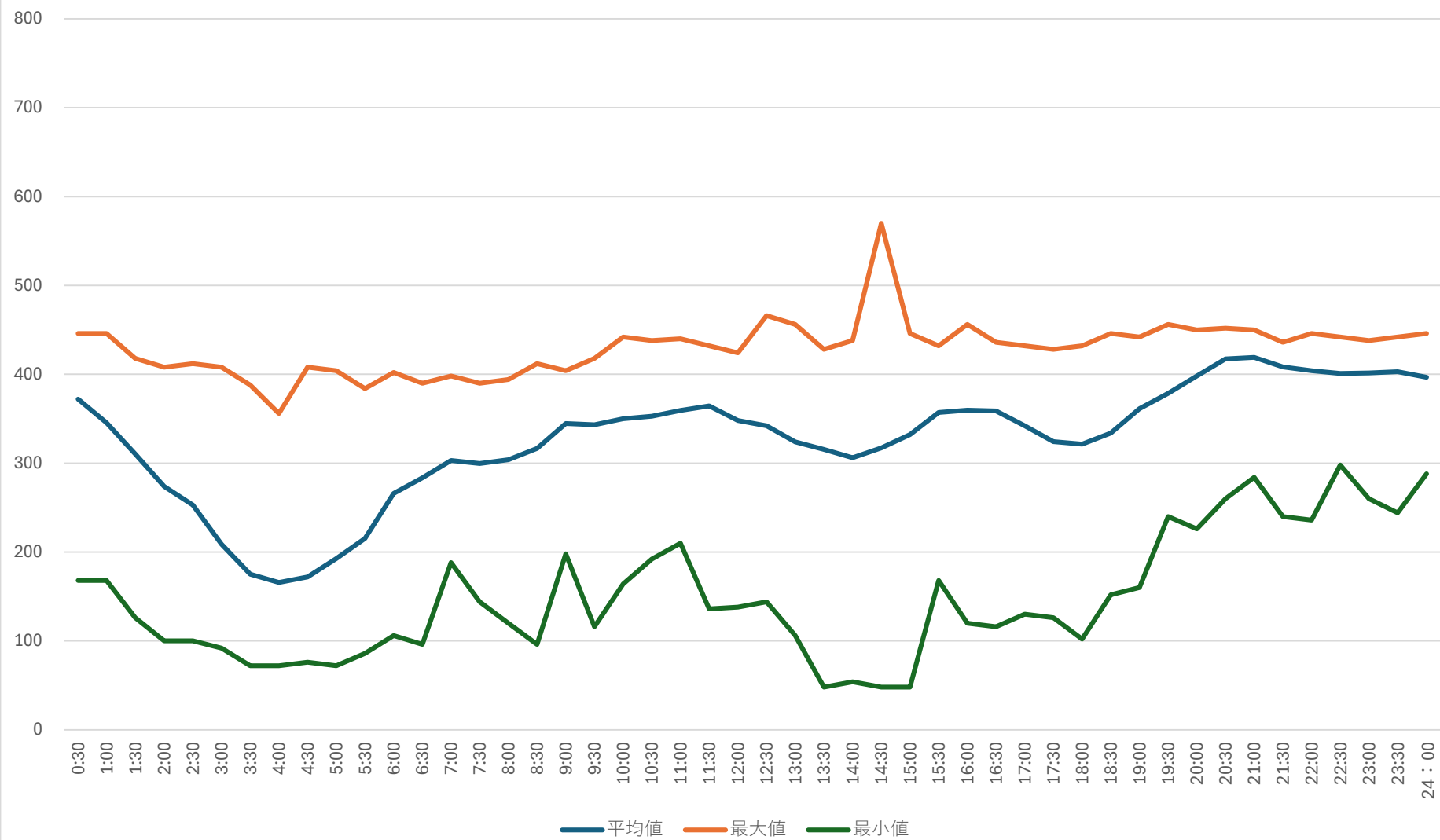
大里浄水場 受電電力量トレンド（11月）
