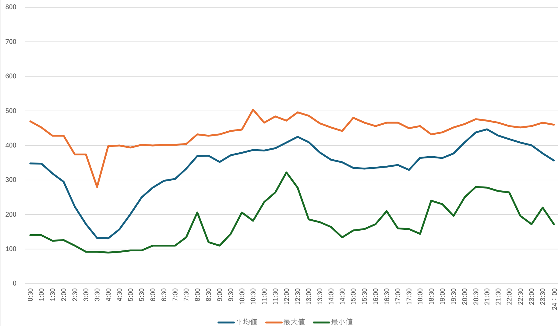
大里浄水場 受電電力量トレンド（7月）
