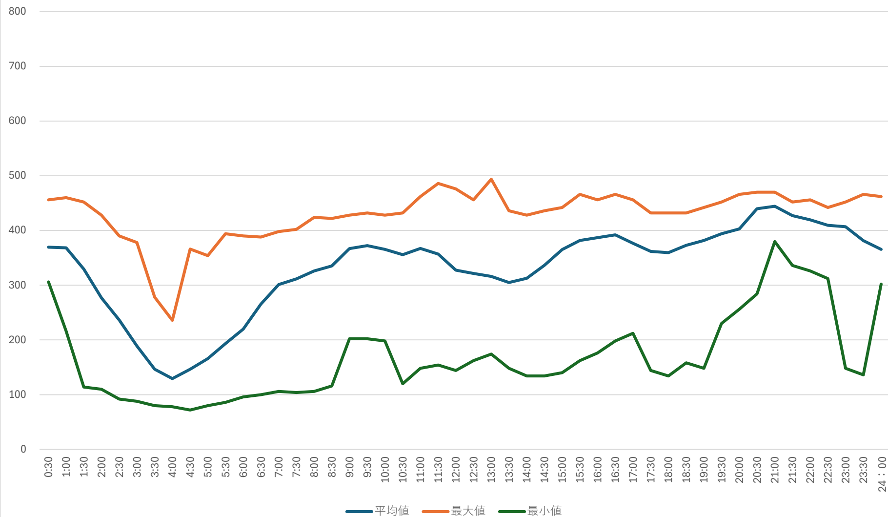
大里浄水場 受電電力量 トレンド（6月）
