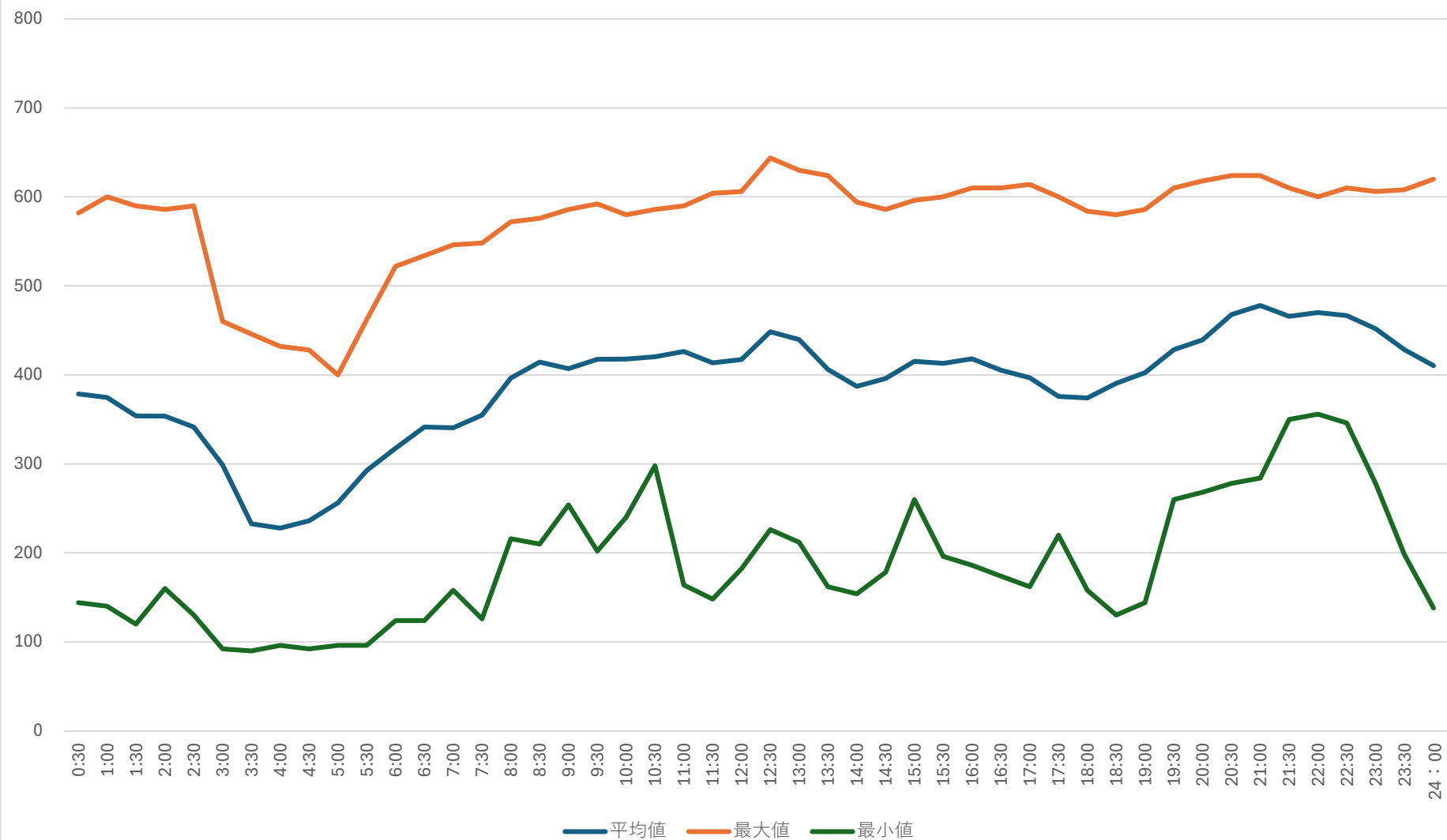
大里浄水場 受電電力量トレンド（8月）
