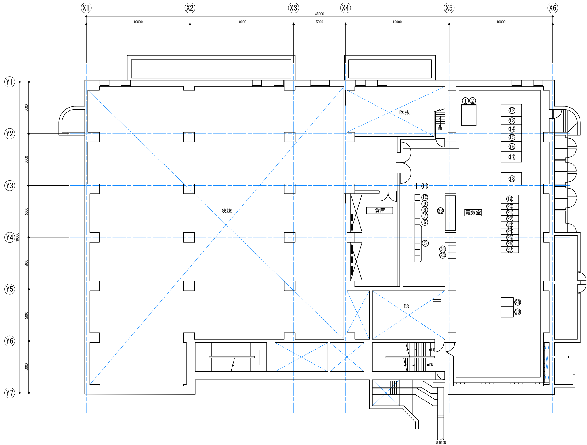
管理本館 地下1階平面図
