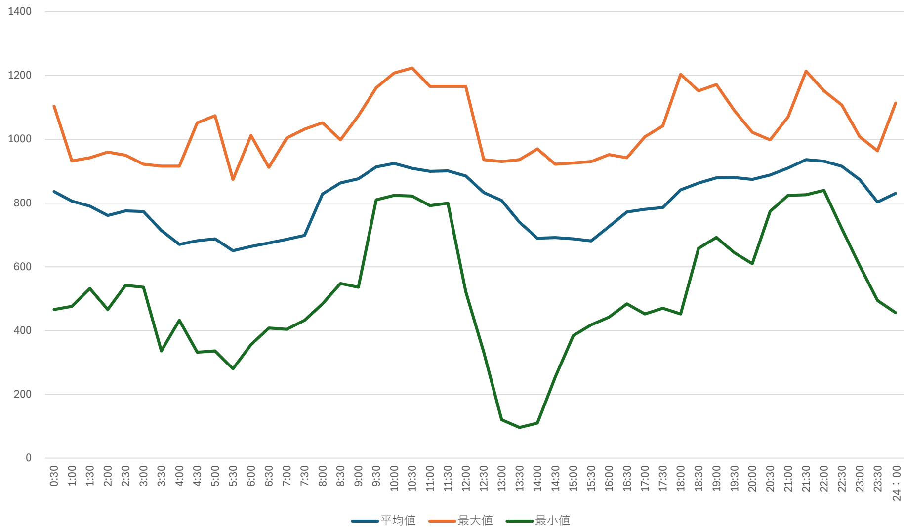
多気浄水場 受電電力量トレンド（1月）
