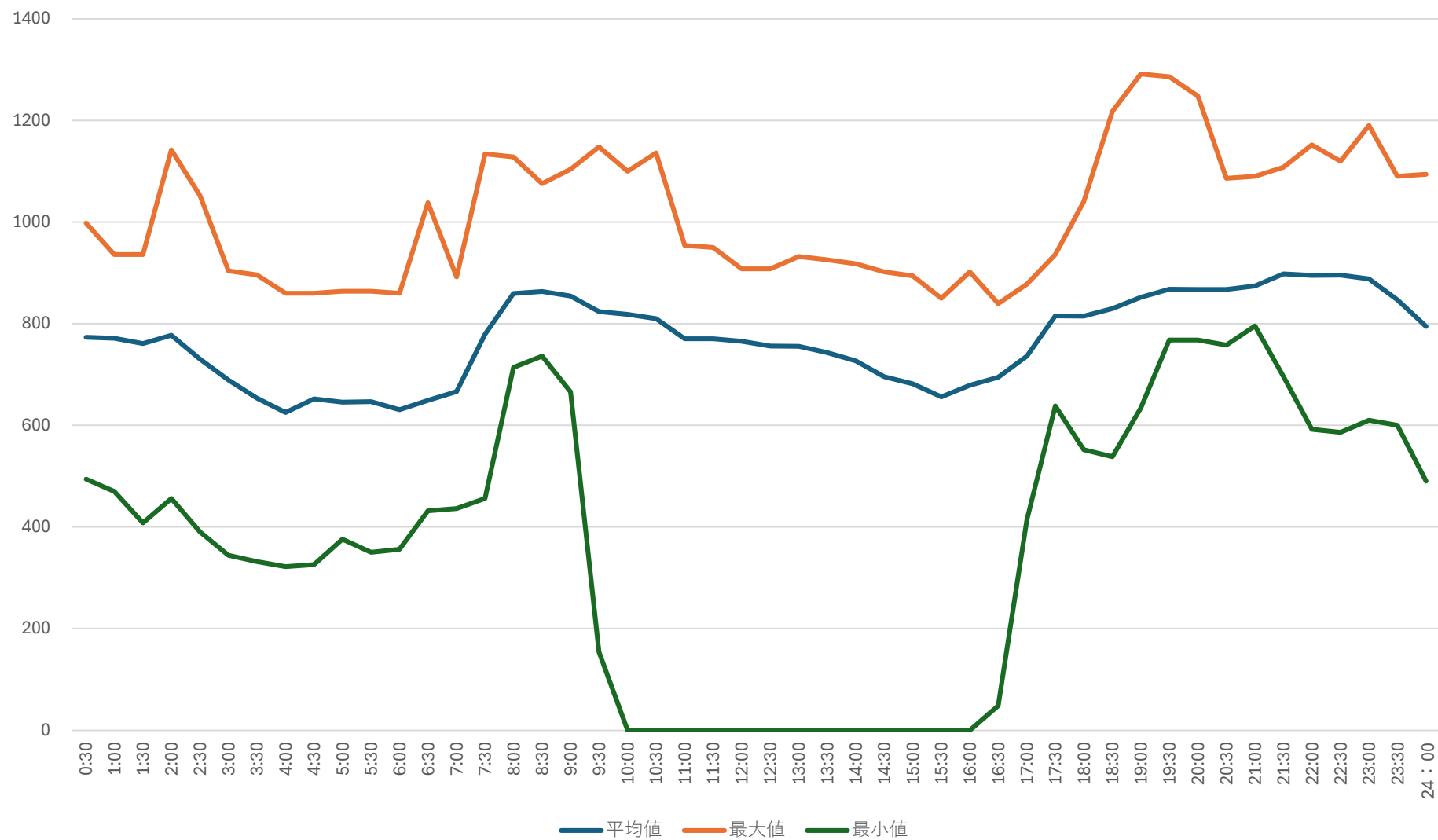
多気浄水場 受電電力量トレンド（12月）
