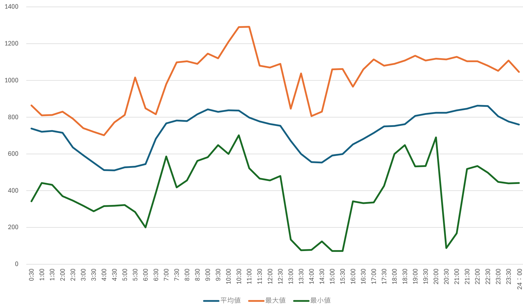
多気浄水場 受電電力量トレンド（9月）
