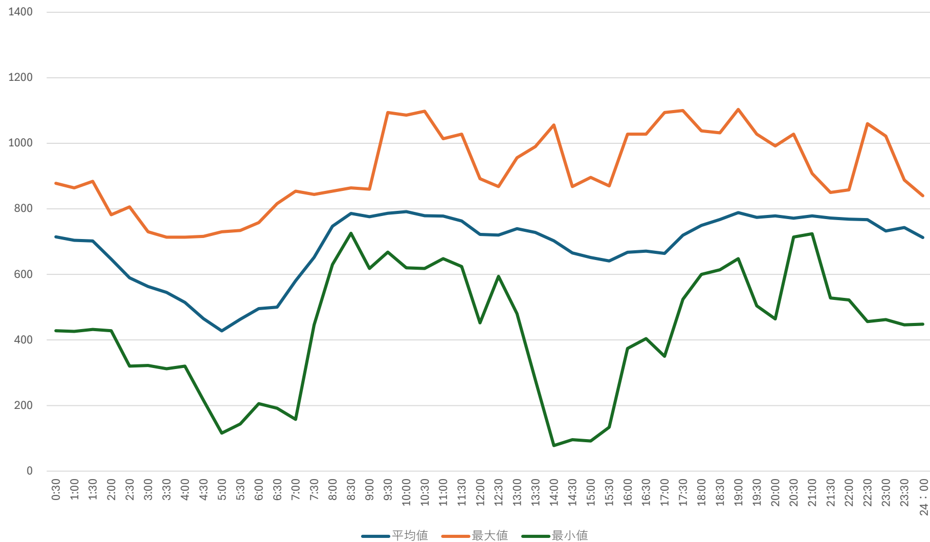
多気浄水場 受電電力量 トレンド（6月）
