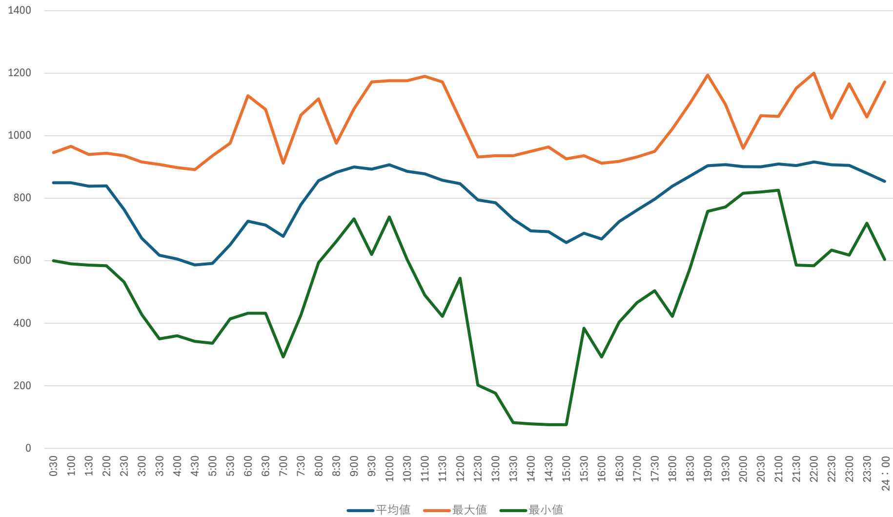
多気浄水場 受電電力量トレンド（2月）
