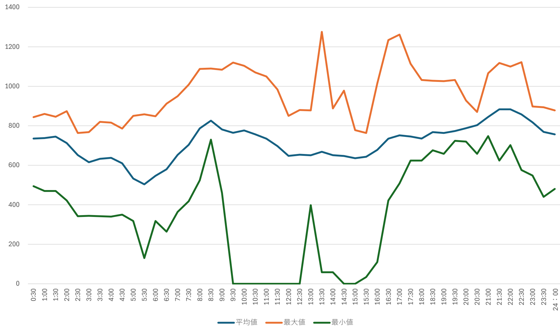
多気浄水場 受電電力量トレンド（11月）
