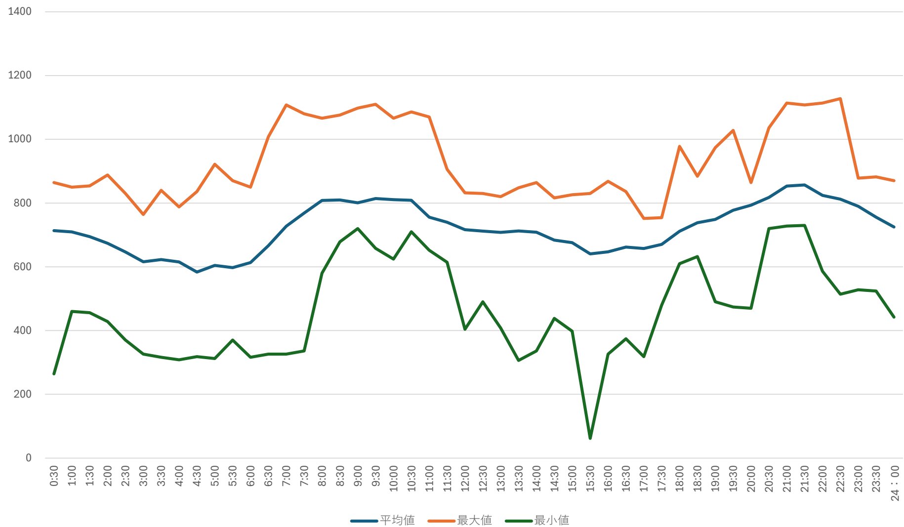
多気浄水場 受電電力量トレンド（10月）
