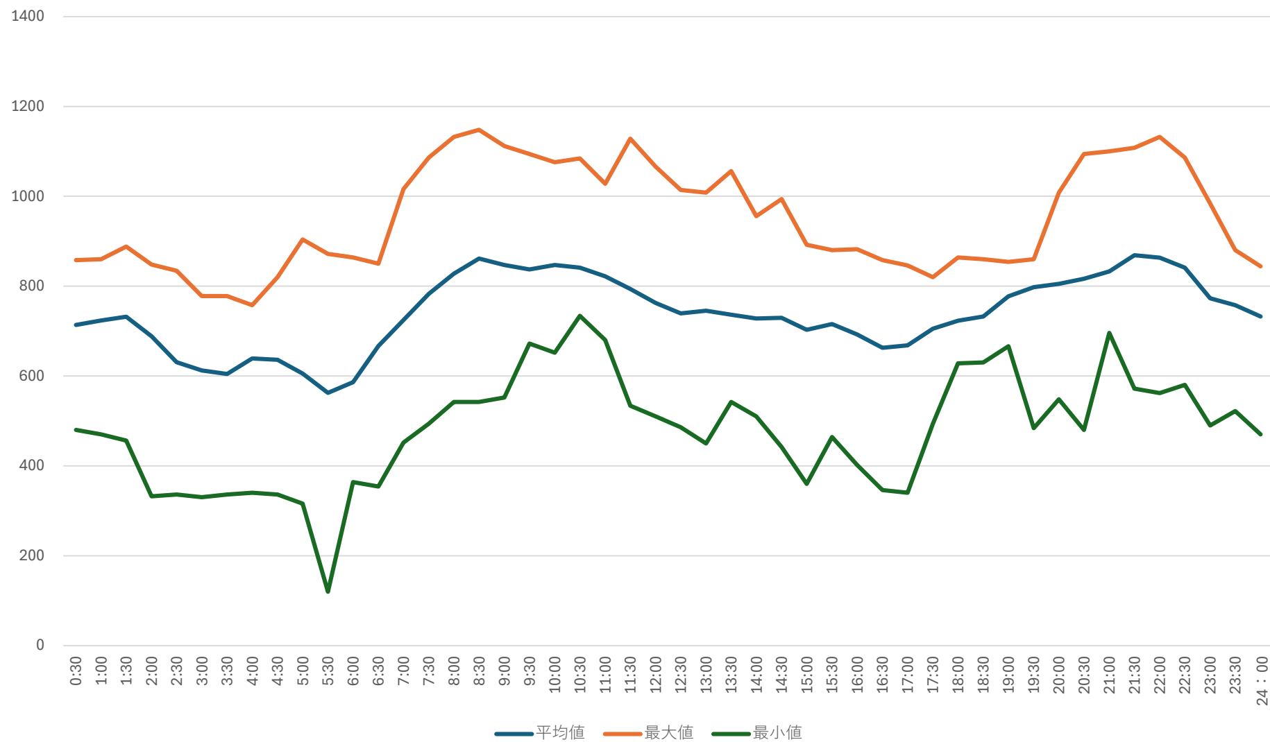
多気浄水場 受電電力量トレンド（7月）
