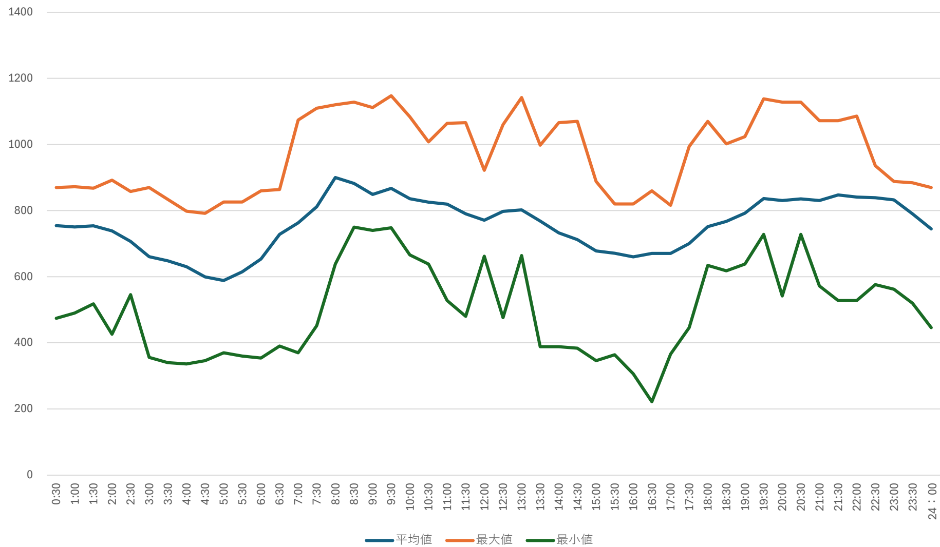
多気浄水場 受電電力量トレンド（8月）
