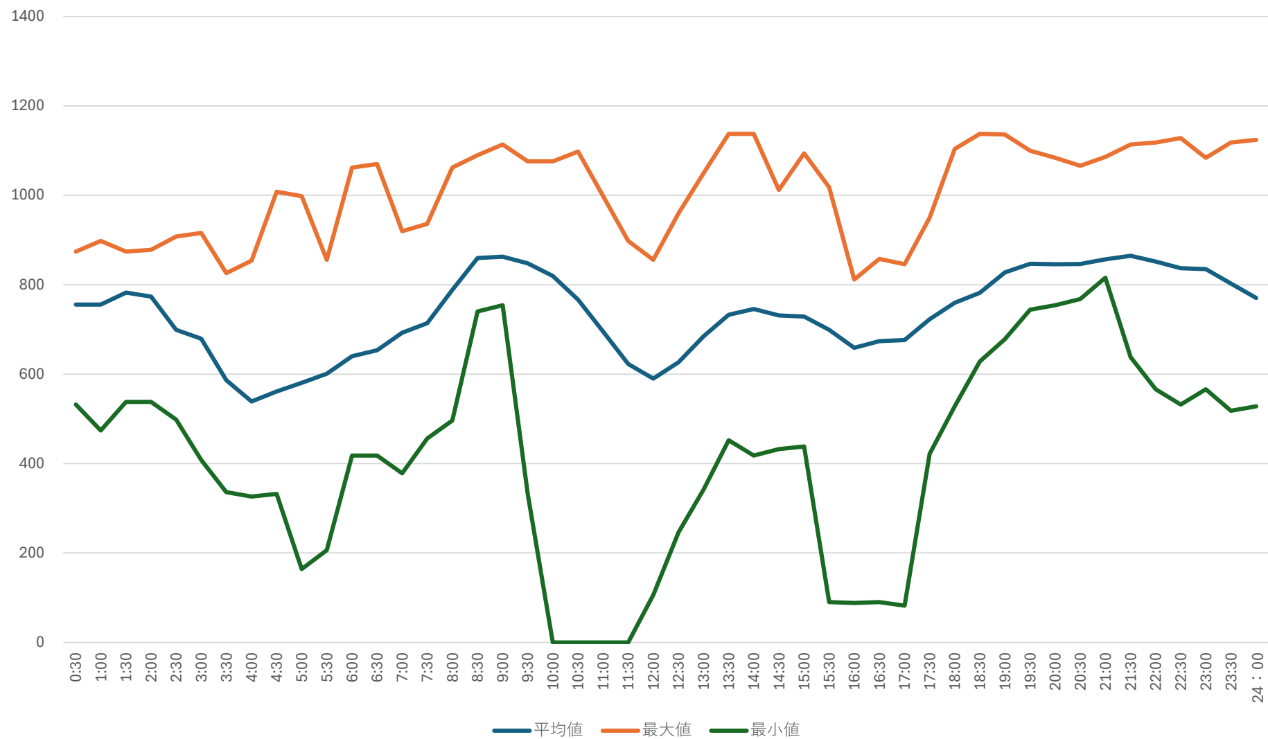
多気浄水場 受電電力量トレンド（3月）
