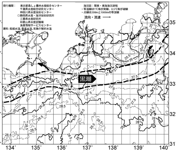
9月17日の海況図
