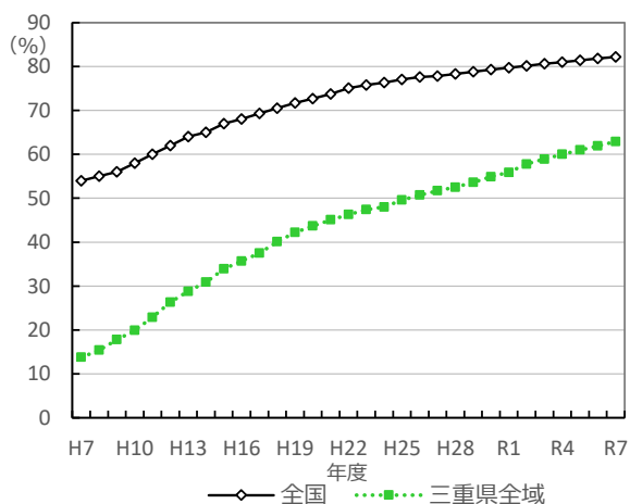
図 2-4-6 下水道普及率の変化
