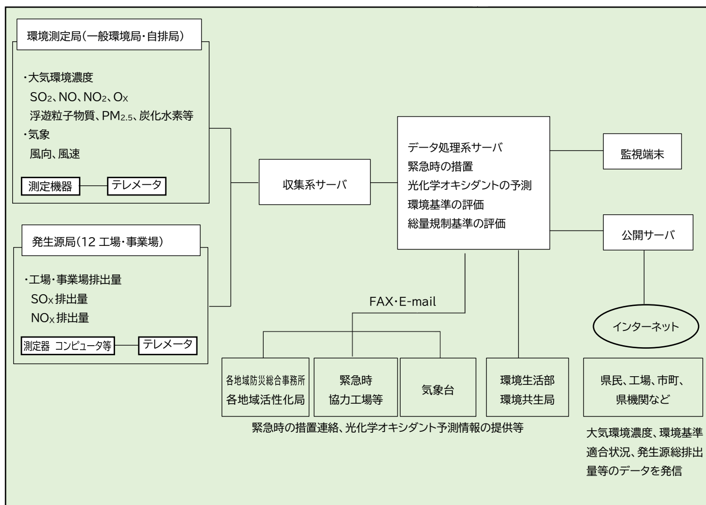
図 2-5-6 環境総合監視システムの概念図
