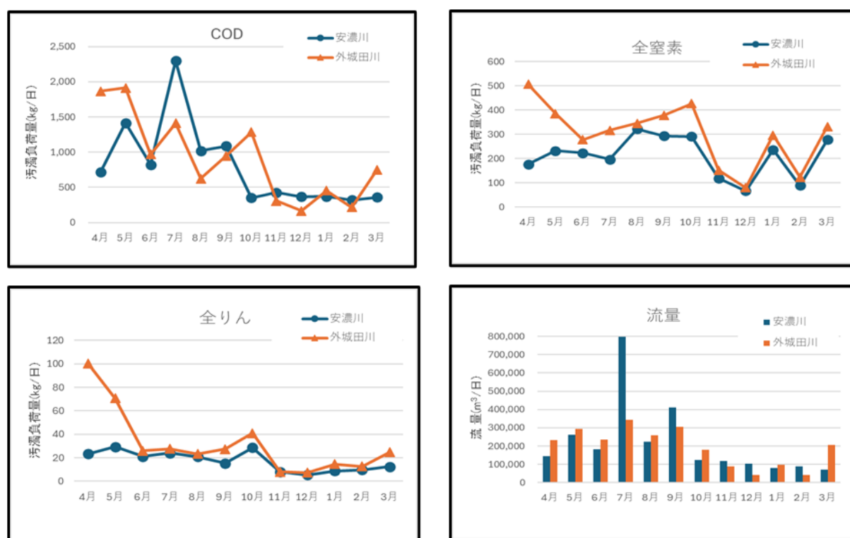
図4 安濃川、外城田川の汚濁負荷量（COD、全窒素、全りん）および流量
