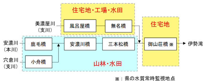
図2 安濃川の調査地点と土地利用状況
