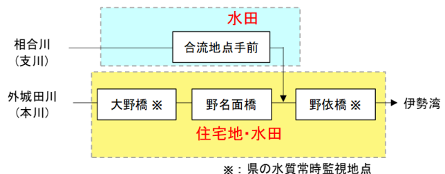
図3 外城田川の調査地点と土地利用状況
