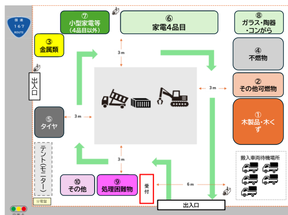
図上演習で選定した仮置場レイアウト図
