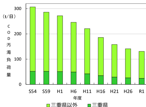
図 2-4-7 伊勢湾の汚濁負荷量の推移 (COD)
