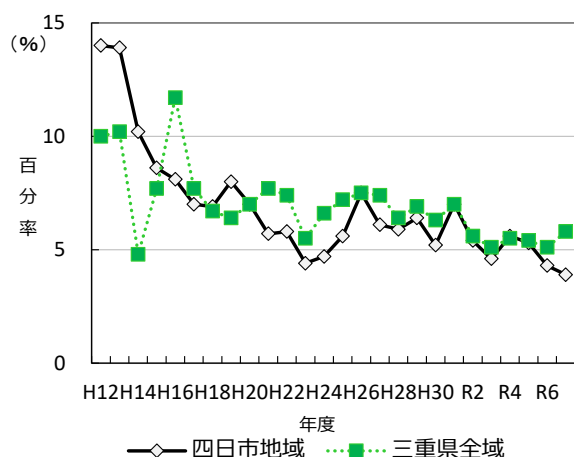
図 2-4-5 光化学オキシダント昼間値（5～20 時）が 0.06ppm を超えた時間数の割合の経年変化
