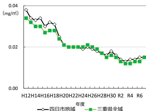
図2-4-3 浮遊粒子状物質の経年変化（一般局の年平均値）
