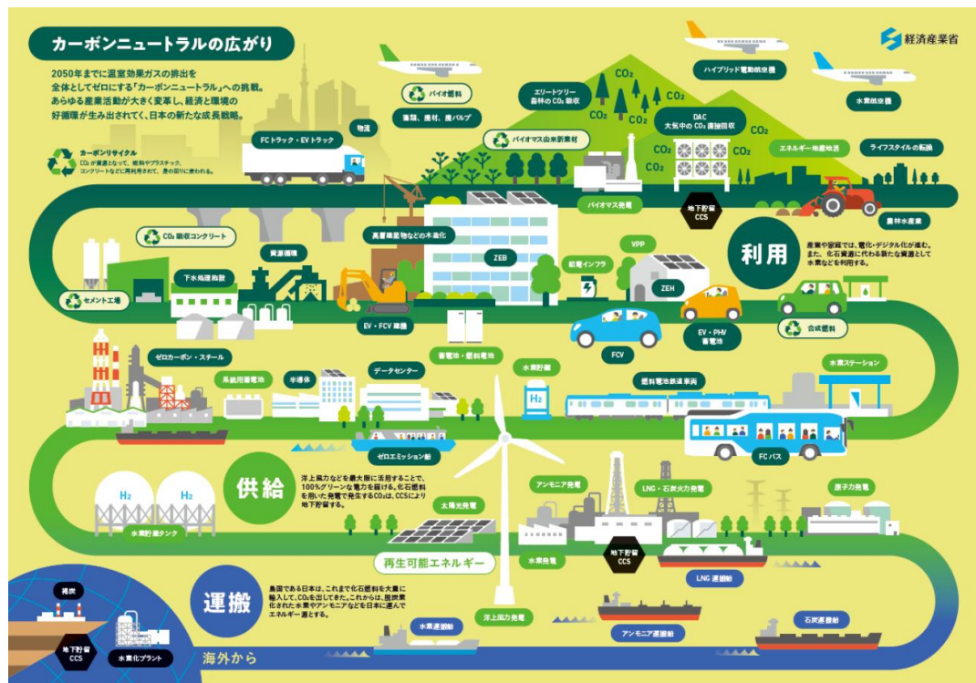
図 2050年カーボンニュートラルに伴うグリーン成長戦略
