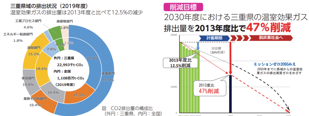
図 温室効果ガスの排出状況及び2030年度における削減目標
