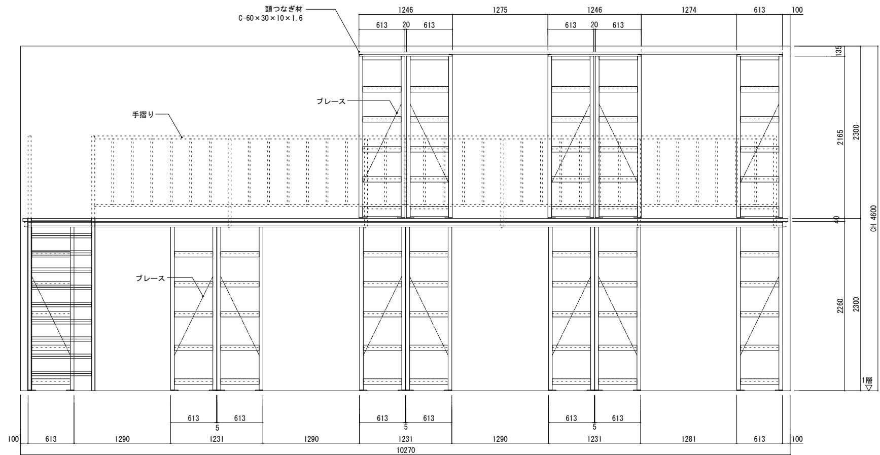
B方向 展開図
