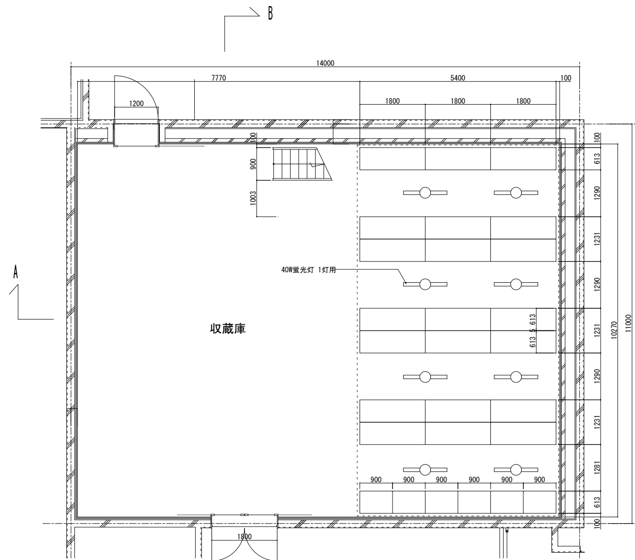
1層平面図 S=1/100
