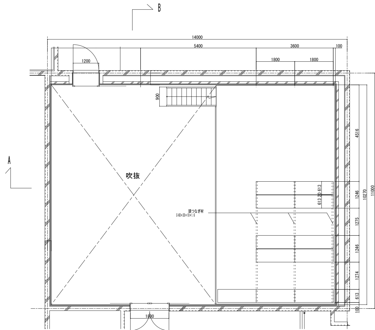
2層平面図 S=1/100
