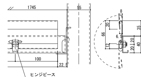
落下防止装置参考詳細図 S=1/5
