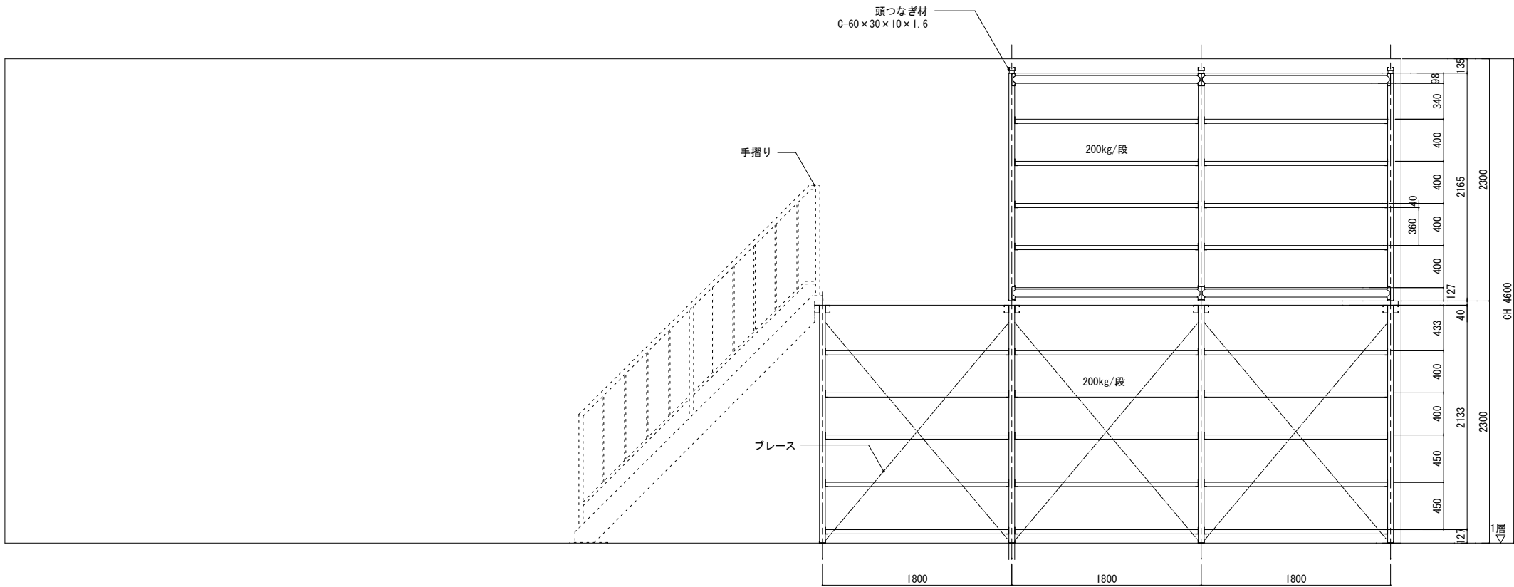
A方向 展開図
