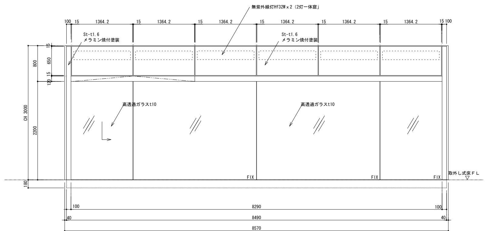
< 壁面展示ケース 展開図 S=1/50>
