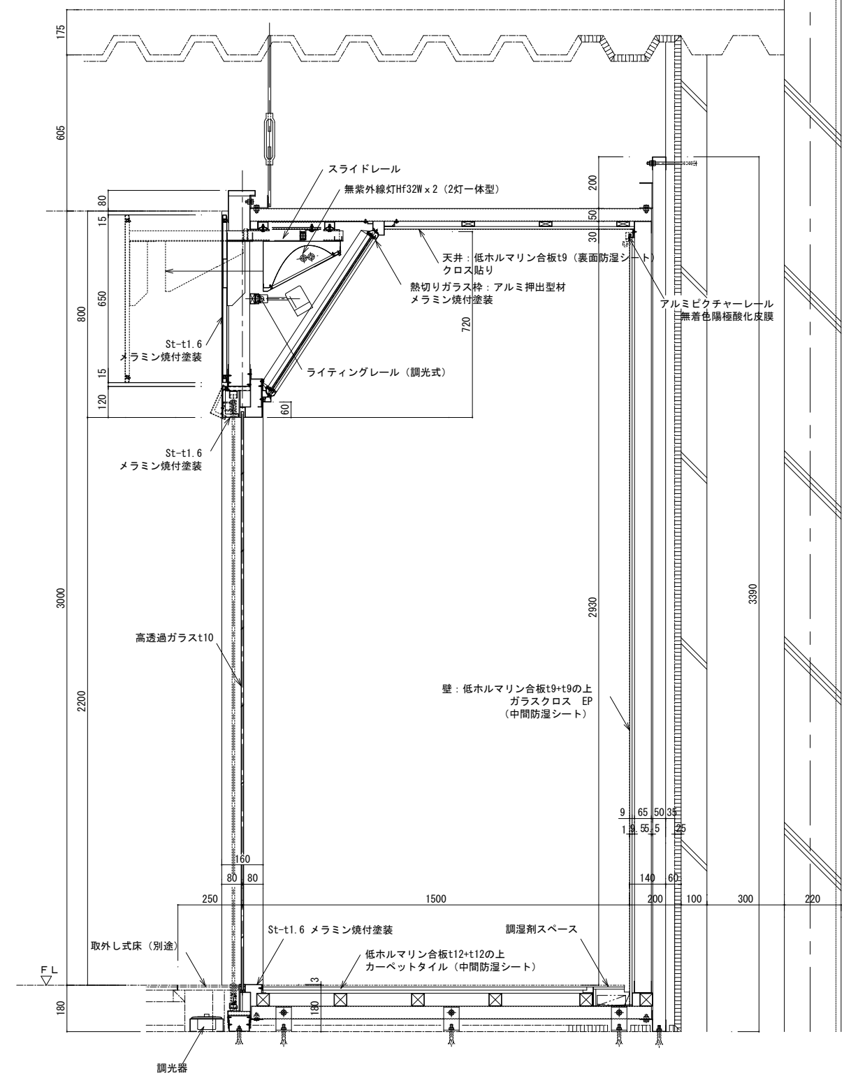
< 壁面展示ケース 主断面図 S=1/20 >
