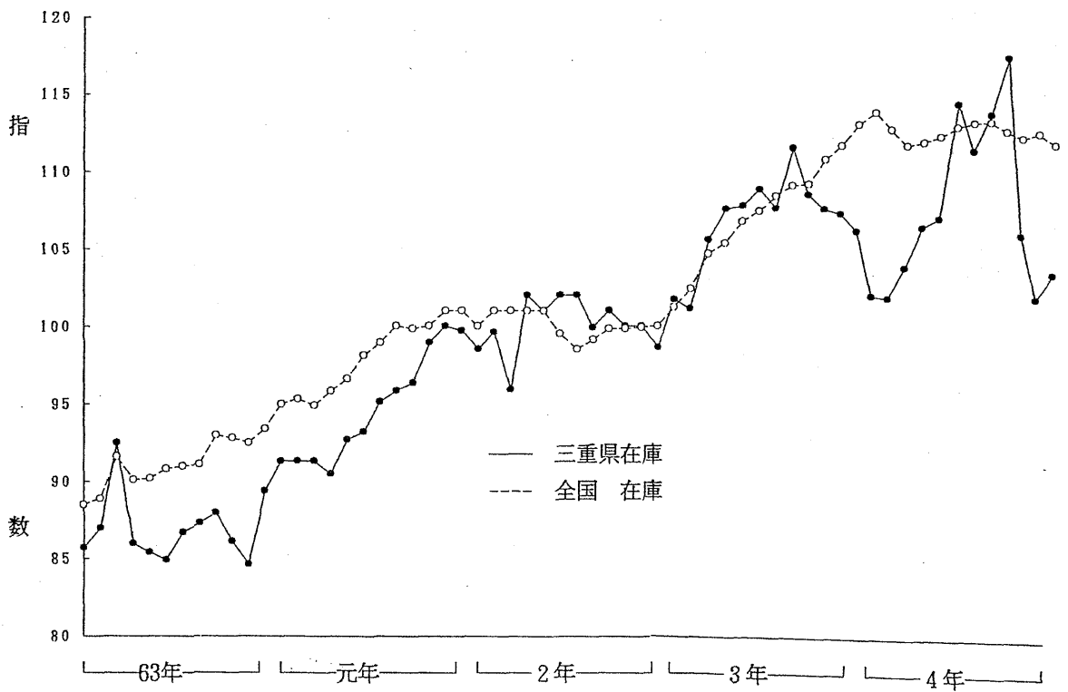
図4 全国・三重県鋳工業生産者製品在庫指数（季節調整済指数）
