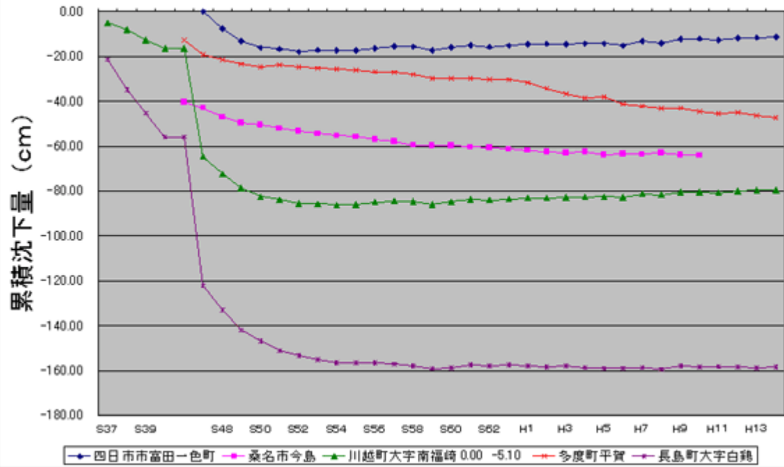
図-1 主な水準点の経年変化
