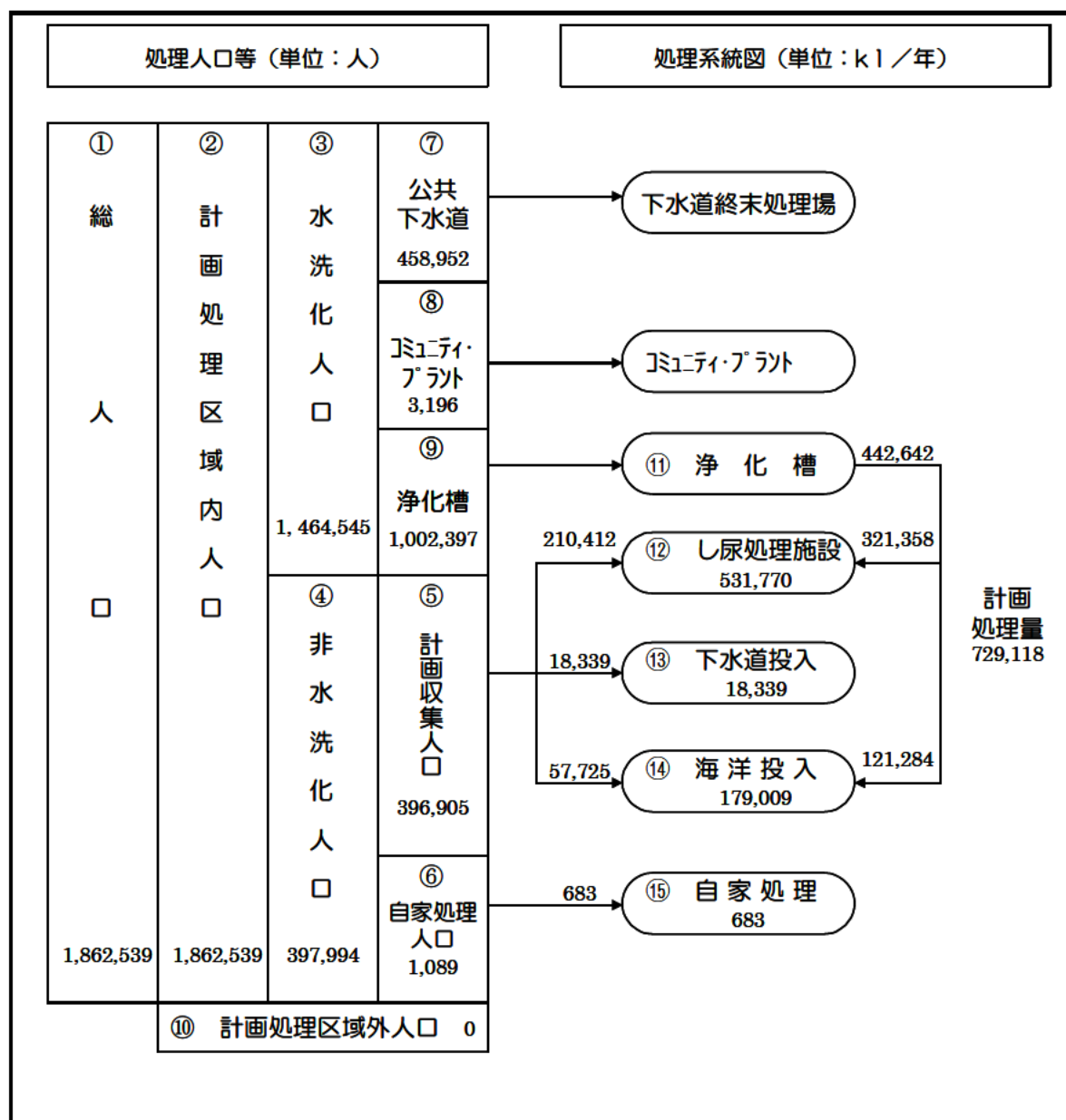
資料7-9 し尿処理のフロー図（平成14年度）
