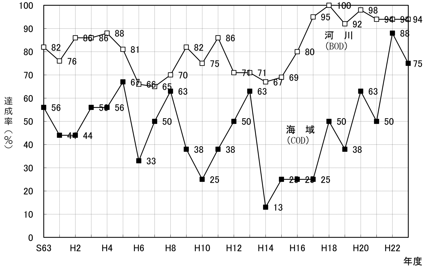
資料3-9 環境基準達成状況の経年変化
