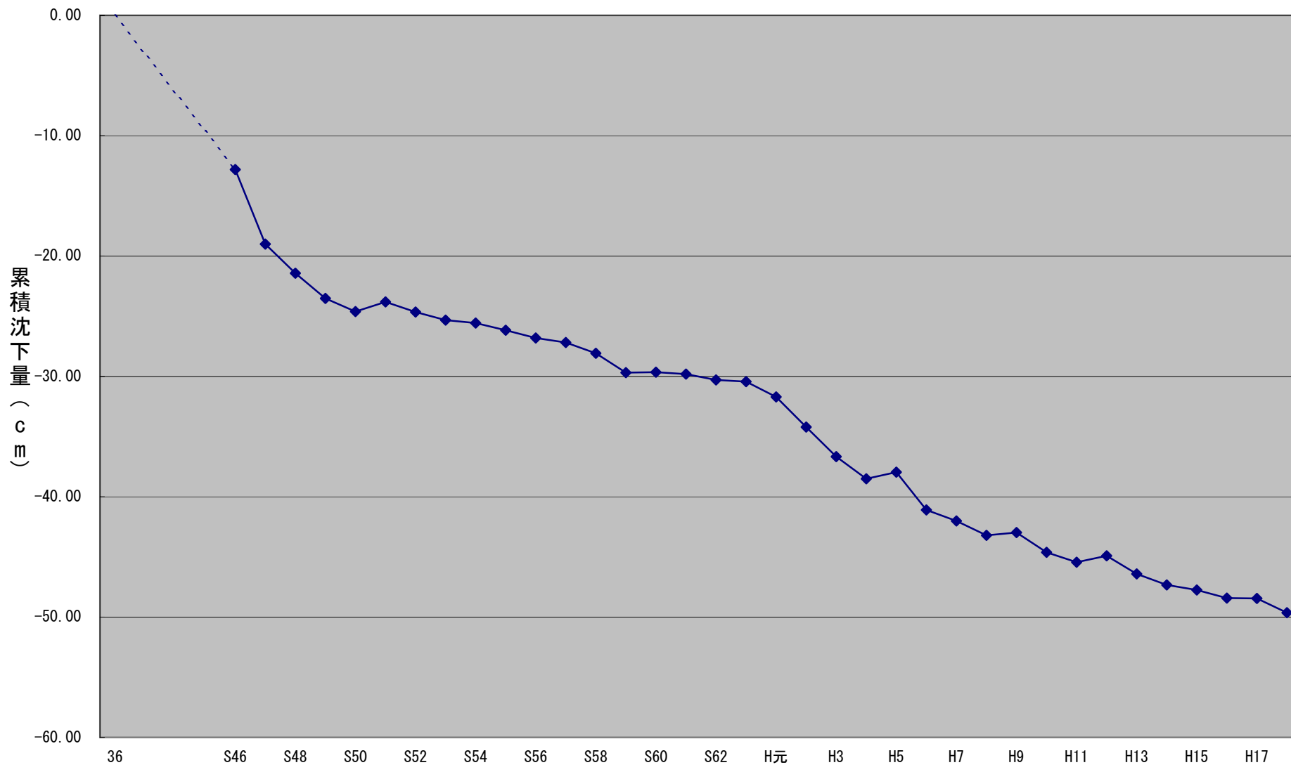
図一3 年間1cm以上の沈下を示した点の経年変化 桑名市多度町福永(平賀)
