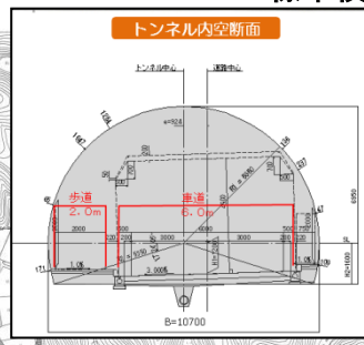
標準横断面図
