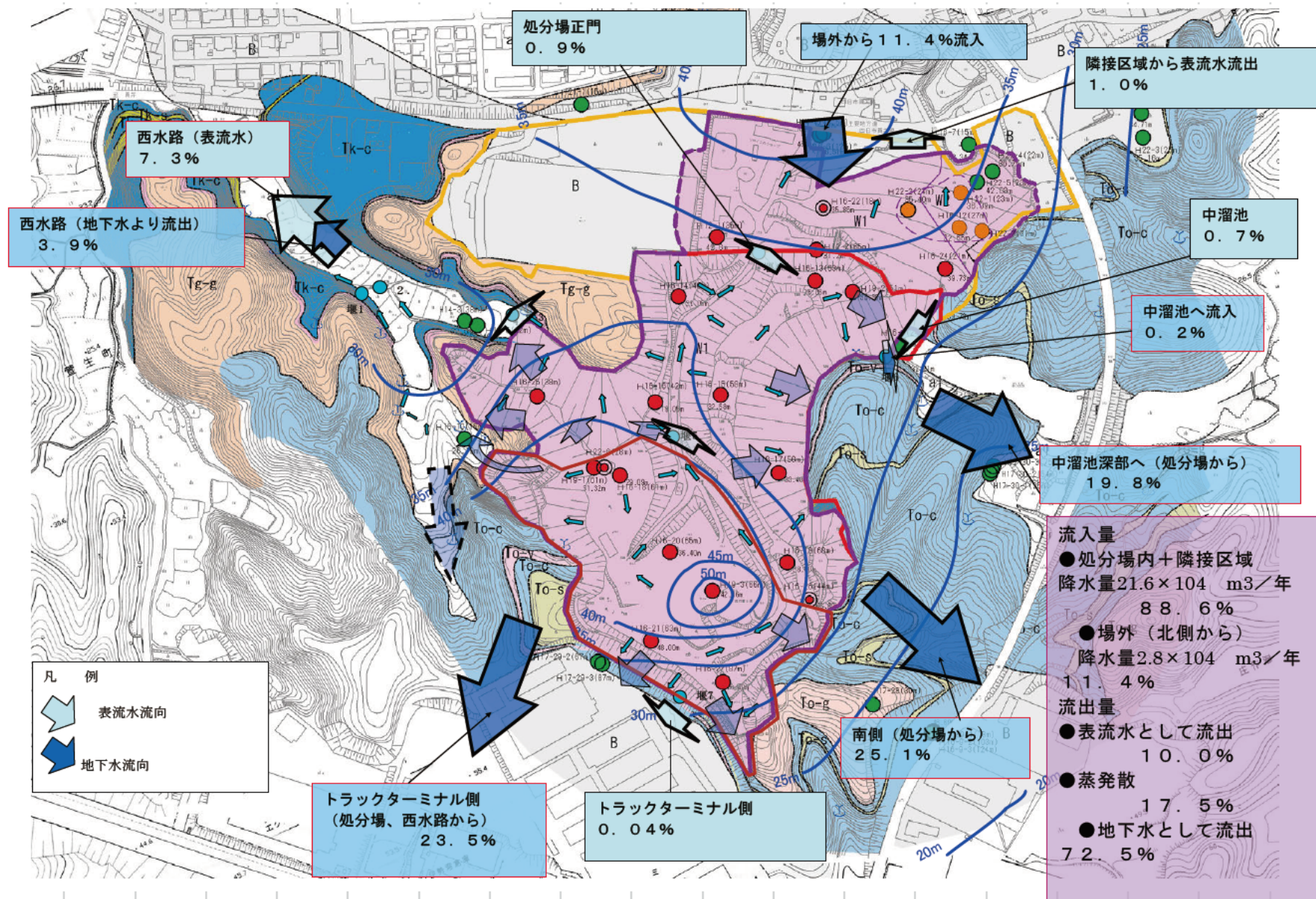
図2-18 地下水等の流向状況解析結果
