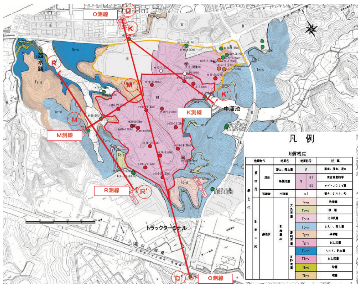
図 2-9 地質平面図
