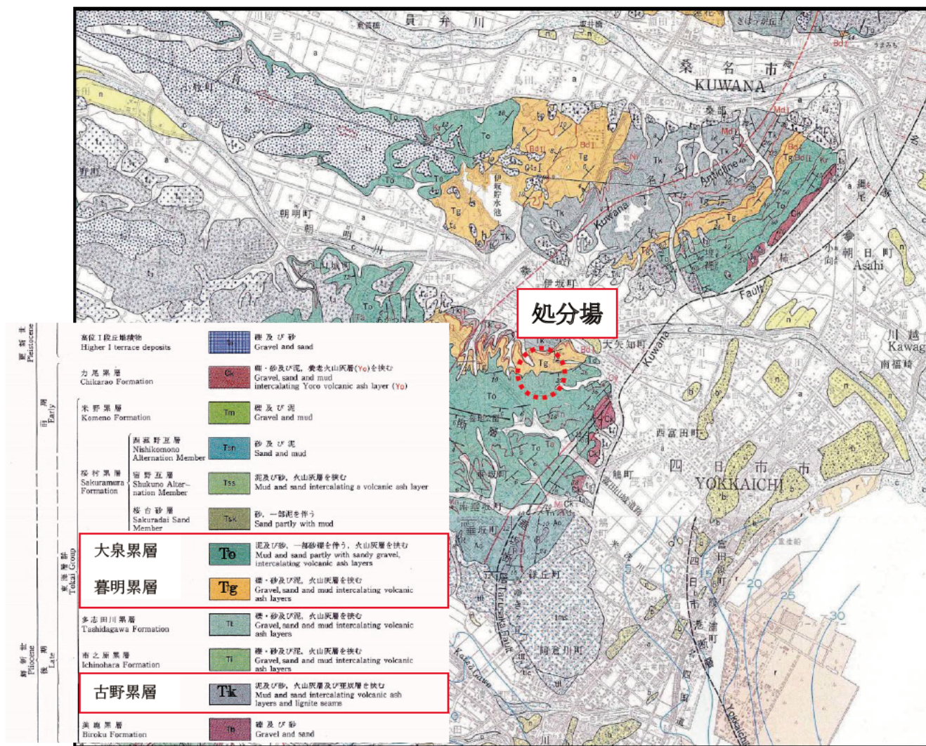
図2-2 広域地質図
