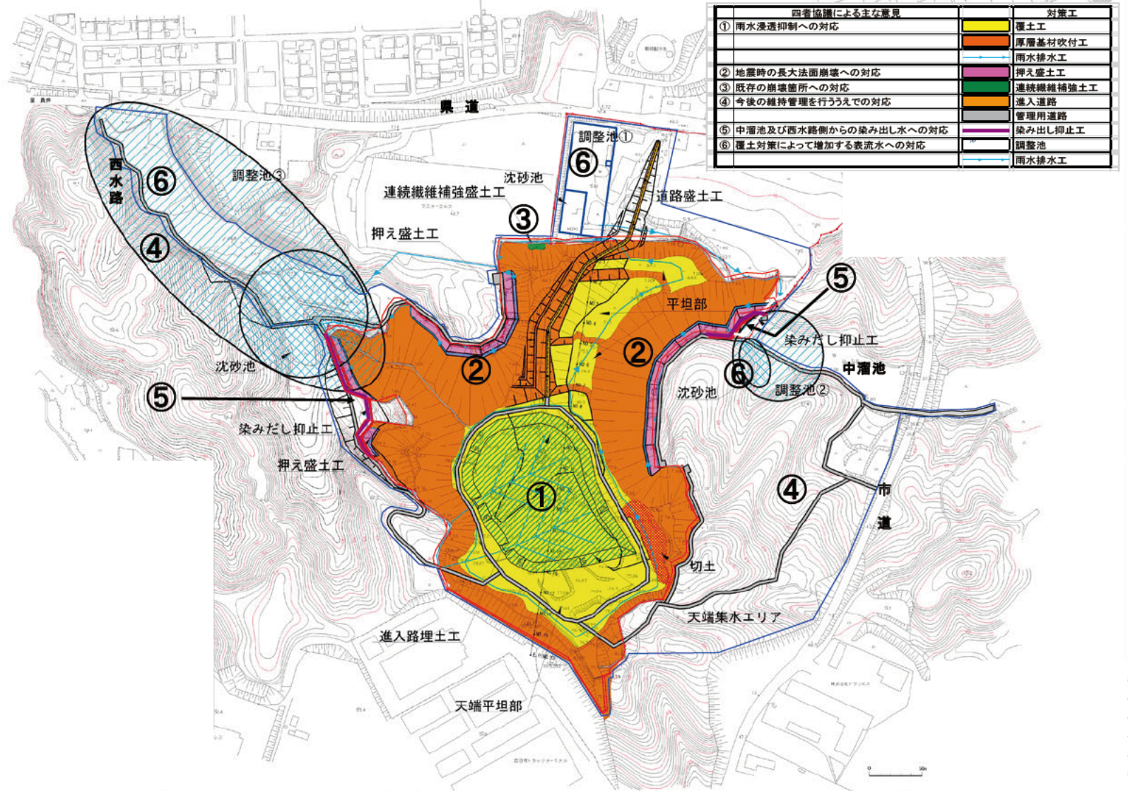
全体計画図(イメージ図) S=1:1000
