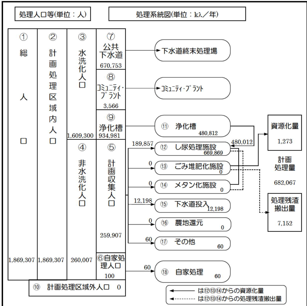
資料7-11 し尿処理のフロー図（平成19年度）
