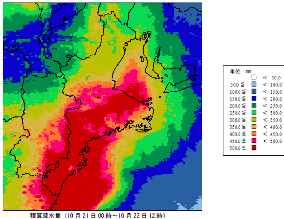
三重県における平成 29 年台風第 21 号の解析雨量による積算降水量
