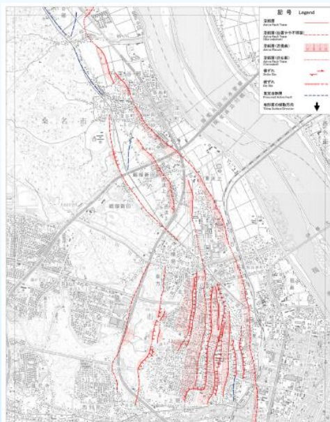
三重県内活断層図
