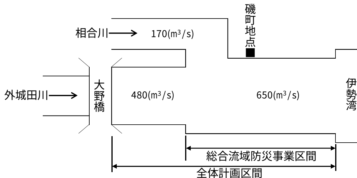
流量配分図
