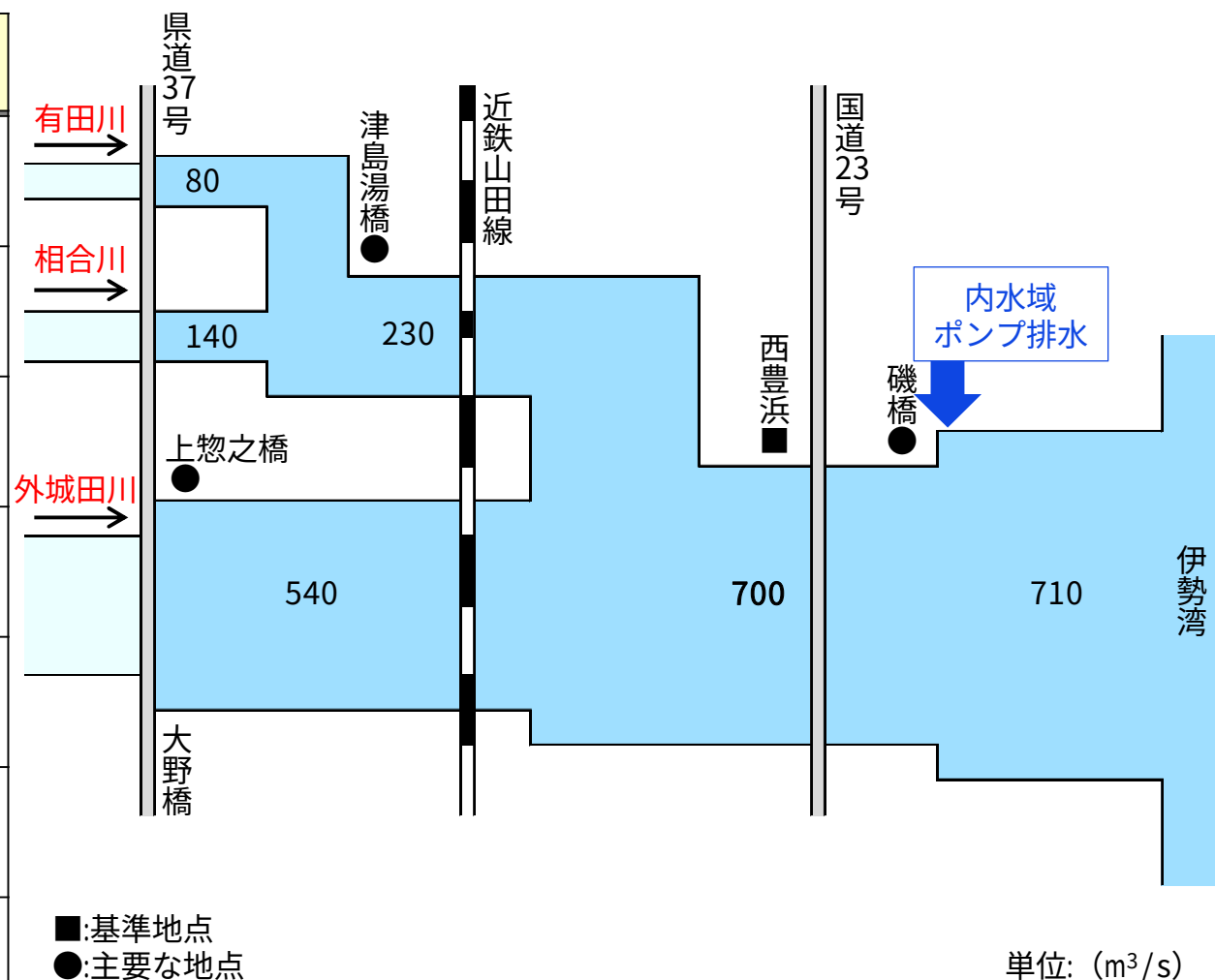
基本高水流量配分図
