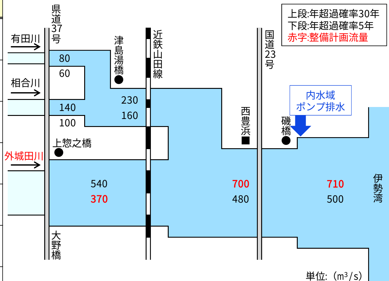
基本高水流量配分図(河川整備計画)
