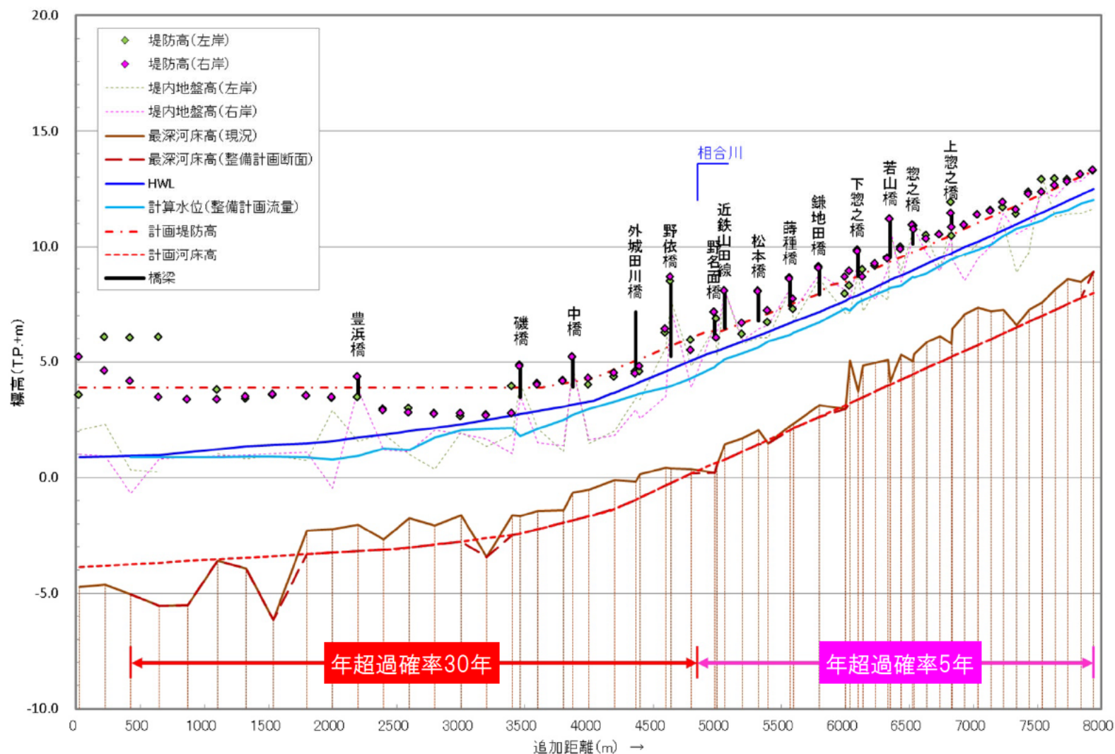
外城田川 水位縦断面図(整備計画断面)
