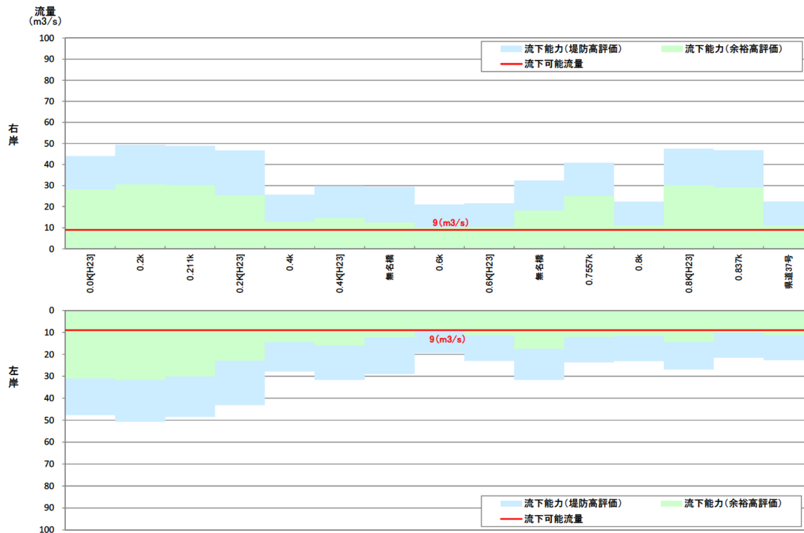
有田川 現況流下能力図
