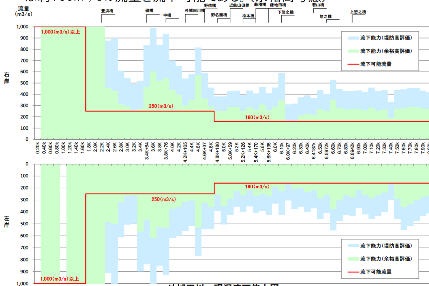
外城田川 現況流下能力図
