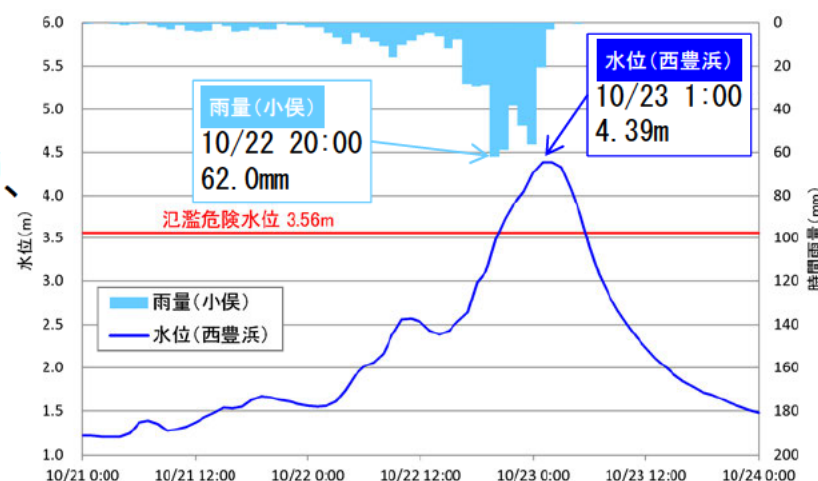
平成29年台風第21号の雨量と水位
