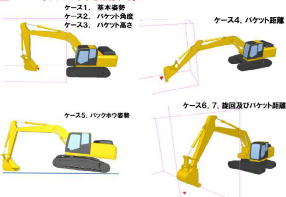
バケット位置精度の確認方法
