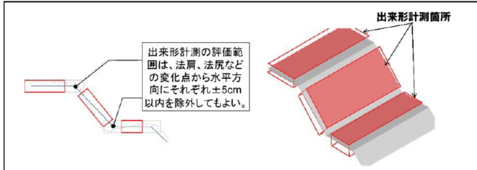
出典：出来形管理要領 4-4 出来形計測箇所 図4-4 出来形計測箇所
