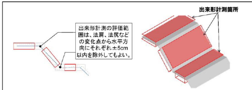
出典：出来形管理要領 4-4 TLSによる出来形計測箇所 図4-4 出来形計測箇所
