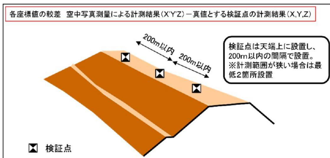
書図-4-1 精度確認試験の配置イメージ図
