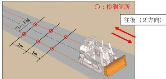
「ブレード位置の取得精度」記録シート (対象技術: ICTブルドーザ)
