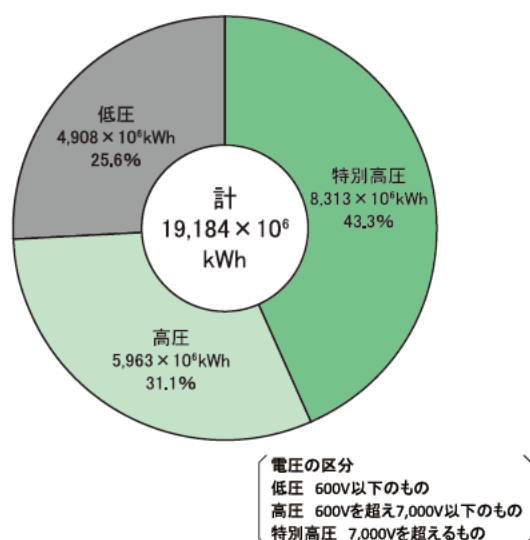
図1-1-4 三重県の電力需要実績（平成29年度）
