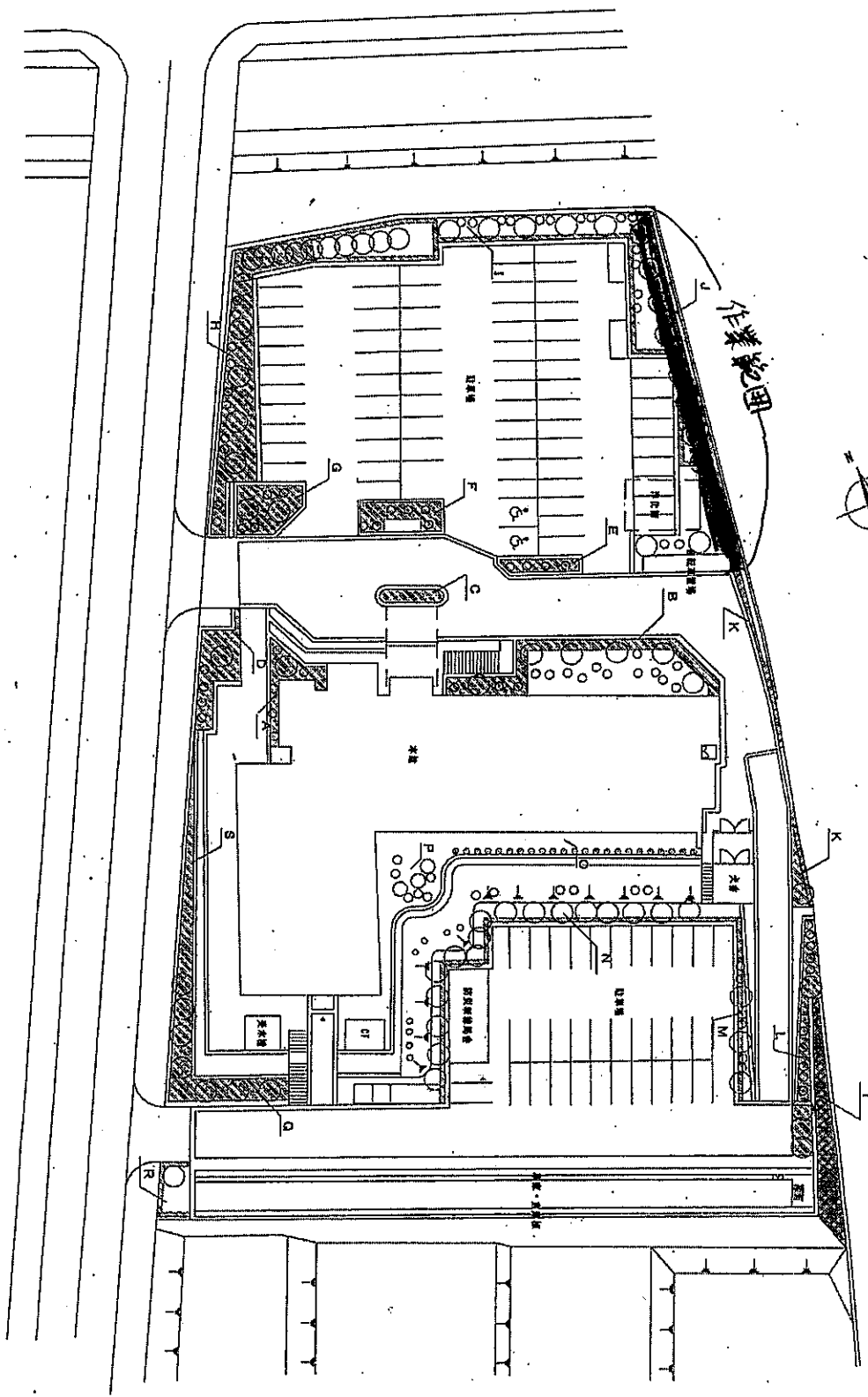
志摩庁舎配置図 1 : 600
