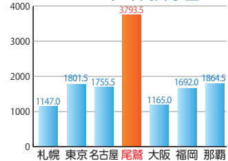
mm/年 2009年 年間降水量
