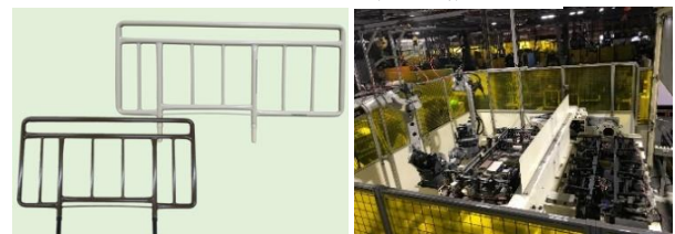
観覧車式溶接ライン
