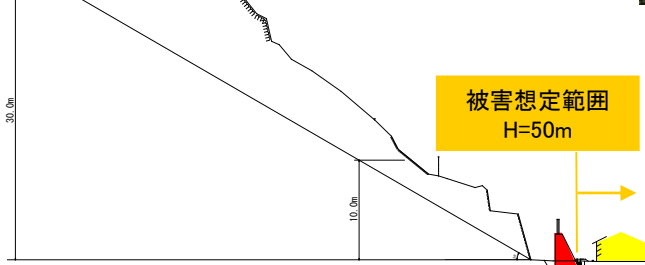
標準断面図
