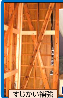
すじかい補強
